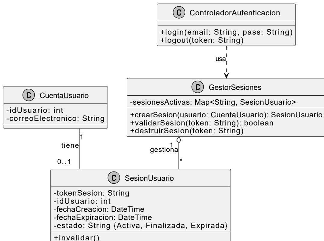
Diagrama de Clases: Proceso de Cierre de Sesión
