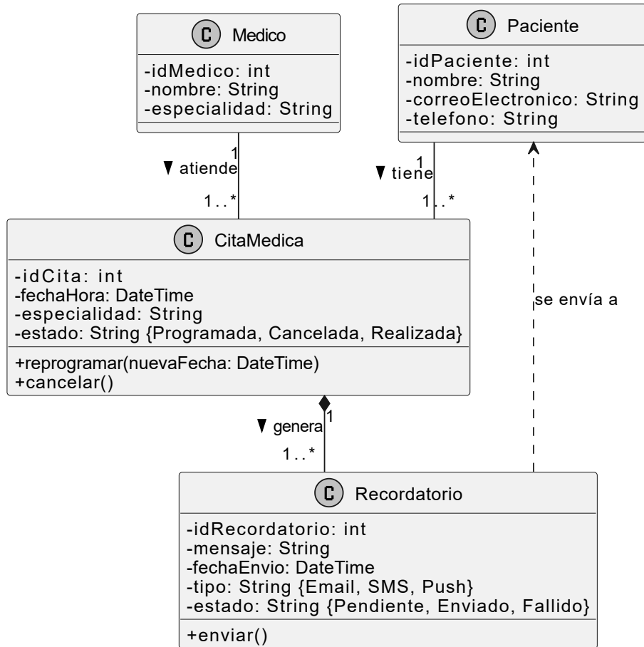
Diagrama de Clases: Sistema de Recordatorios de Citas Médicas
