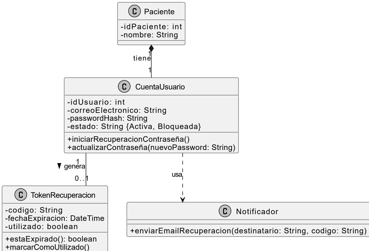
Diagrama de Clases: Proceso de Recuperación de Contraseña
