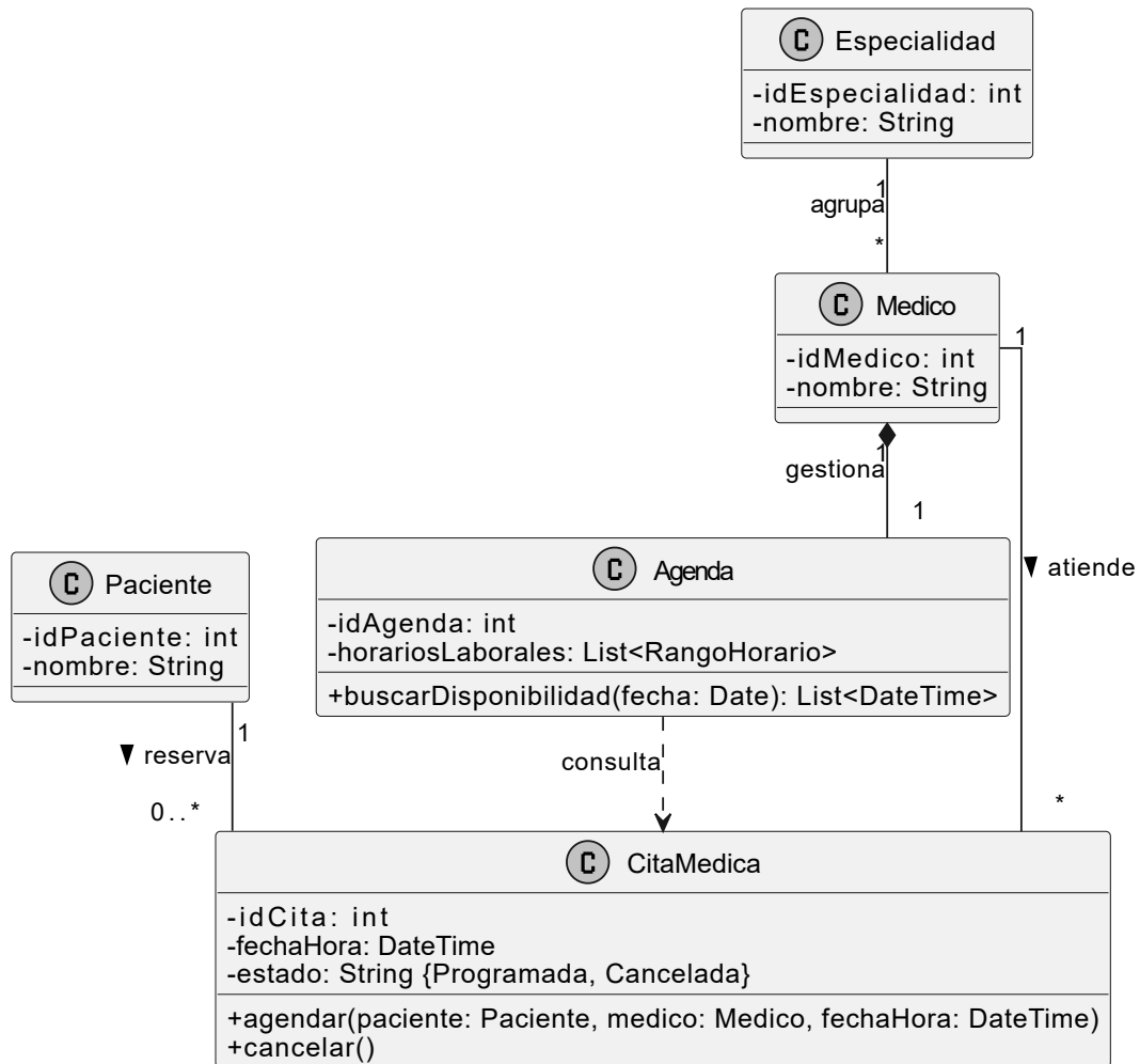
Diagrama de Clases: Visualización y Agendamiento de Citas
