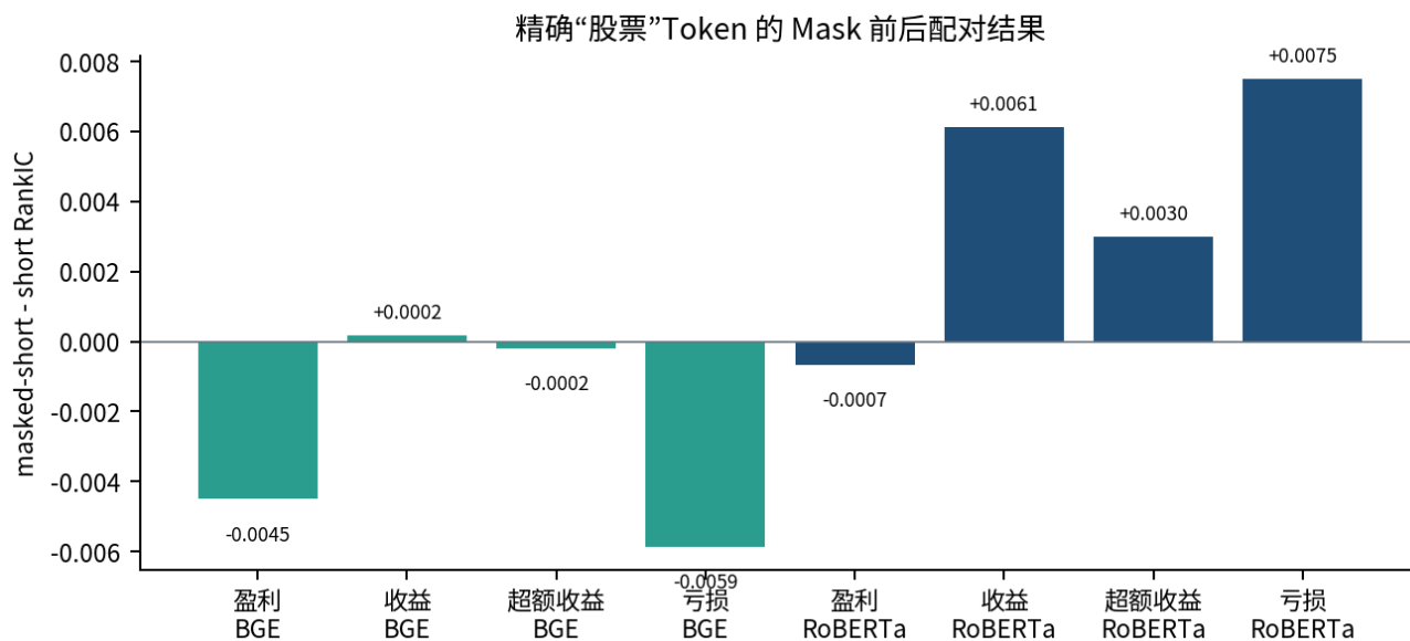
图 4. 精确“股票”Token 的 masked-short 减 short；颜色区分 RoBERTa 与 BGE-M3，正负方向并不一致。
