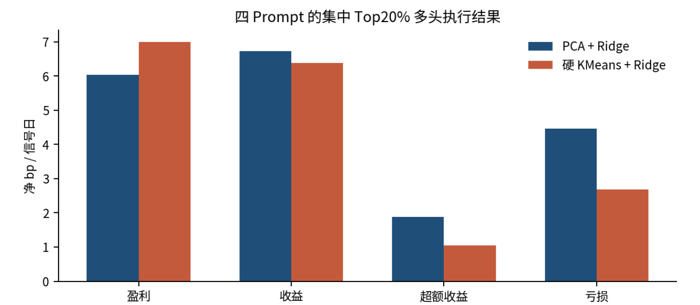
图 4. 相同四 Prompt 的模型和 mask 配对下的 Top20% 多头净 bp；成本已扣，但组合平均仅 2.80 只。
