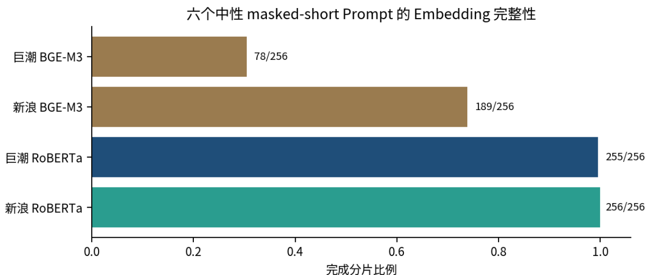
图 6. 中性六 Prompt embedding 分片完成度。未完成 BGE-M3 不能冒充全量结果。
