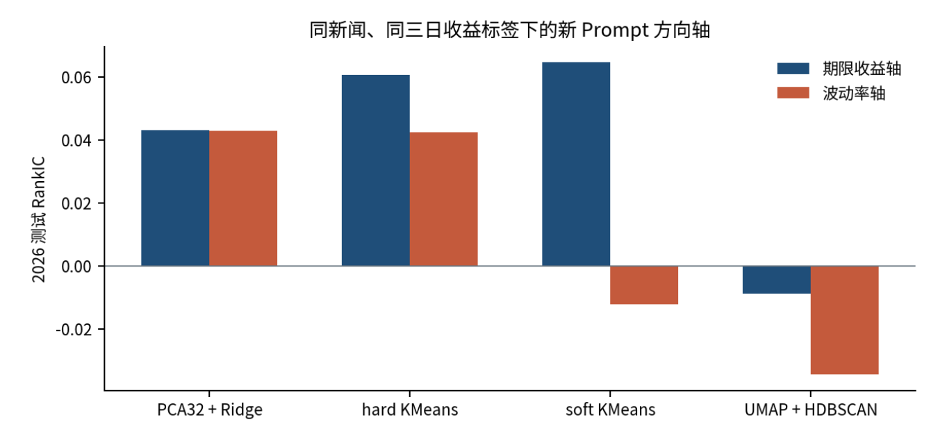
图 4. 同新闻、同三日收益标签下，期限收益轴与波动率轴的 2026 样本外 RankIC \cap
