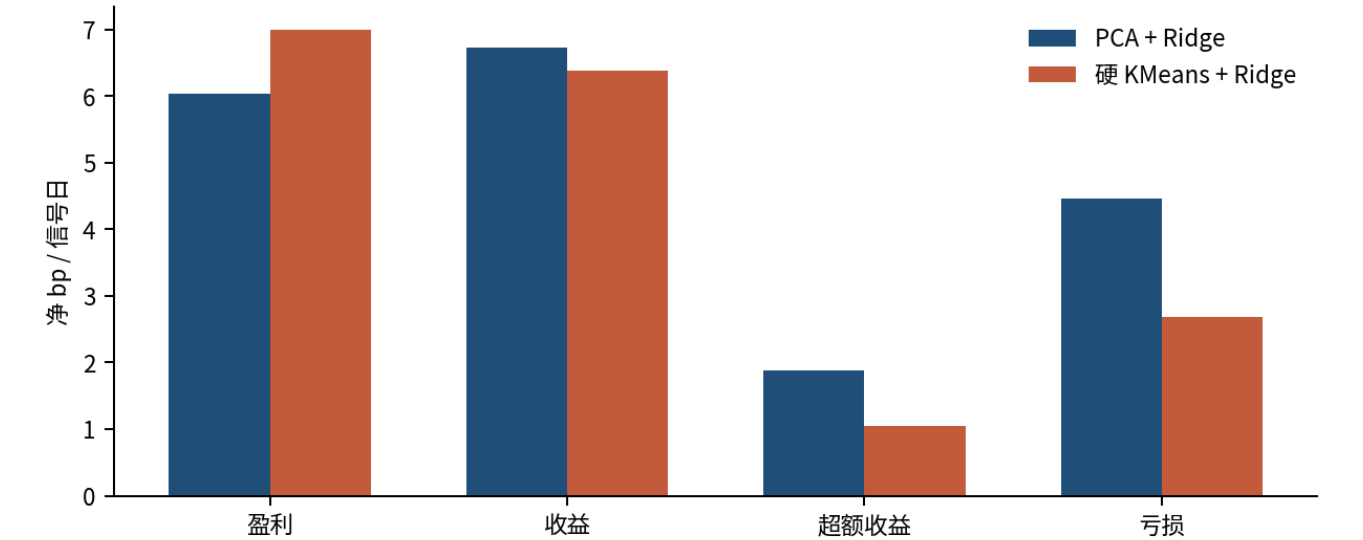
四 Prompt 的集中 Top20% 多头执行结果
