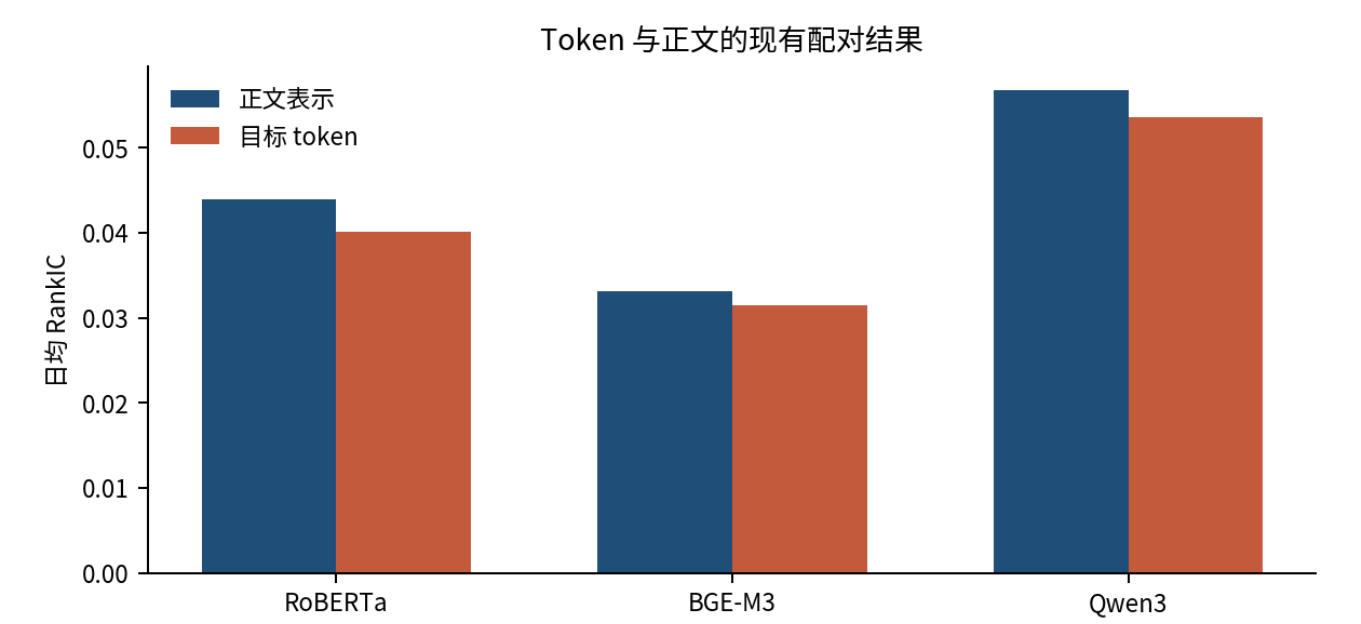
图 3. 三模型现有 token/body 结果。RoBERTa/BGE-M3 是四 Prompt 汇总，Qwen 是单一“收益”Prompt，不能当作完全公平的模型排名。
