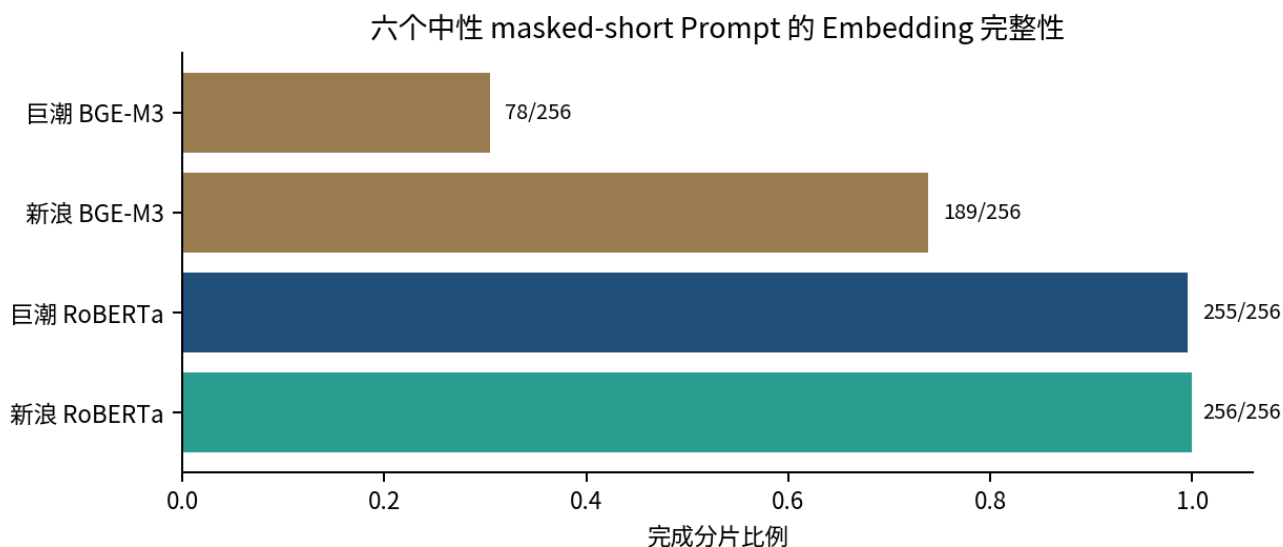
图 4. 中性六 Prompt embedding 分片完成度。未完成 BGE-M3 不能冒充全量结果。
