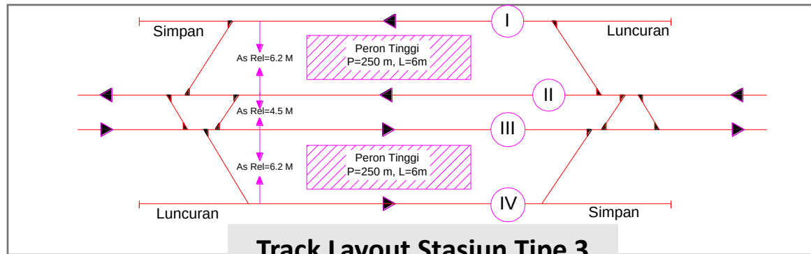
Track Layout Stasiun Tipe 3
