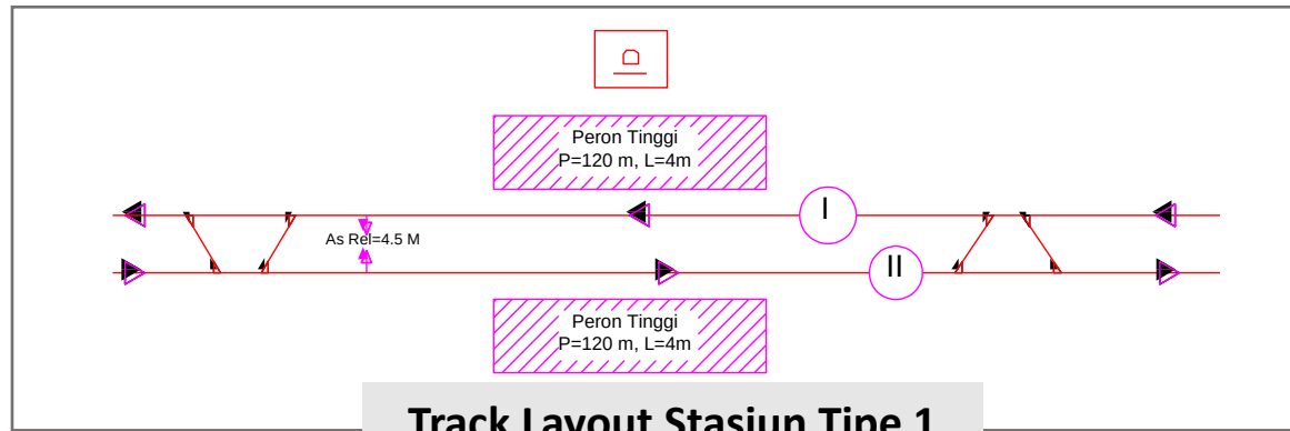
Track Layout Stasiun Tipe 1
