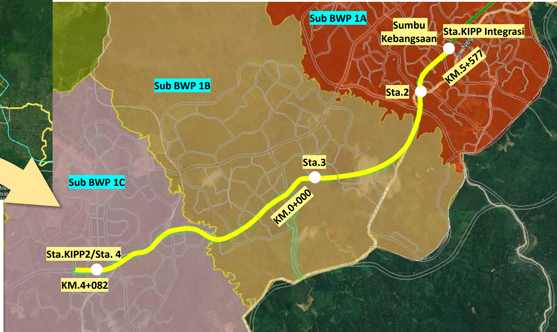
Rencana Jalur KA dan Jalan Arteri Sekunder di KIPP
