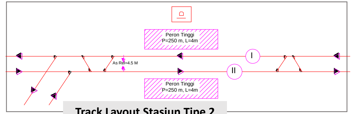
Track Layout Stasiun Tipe 2
