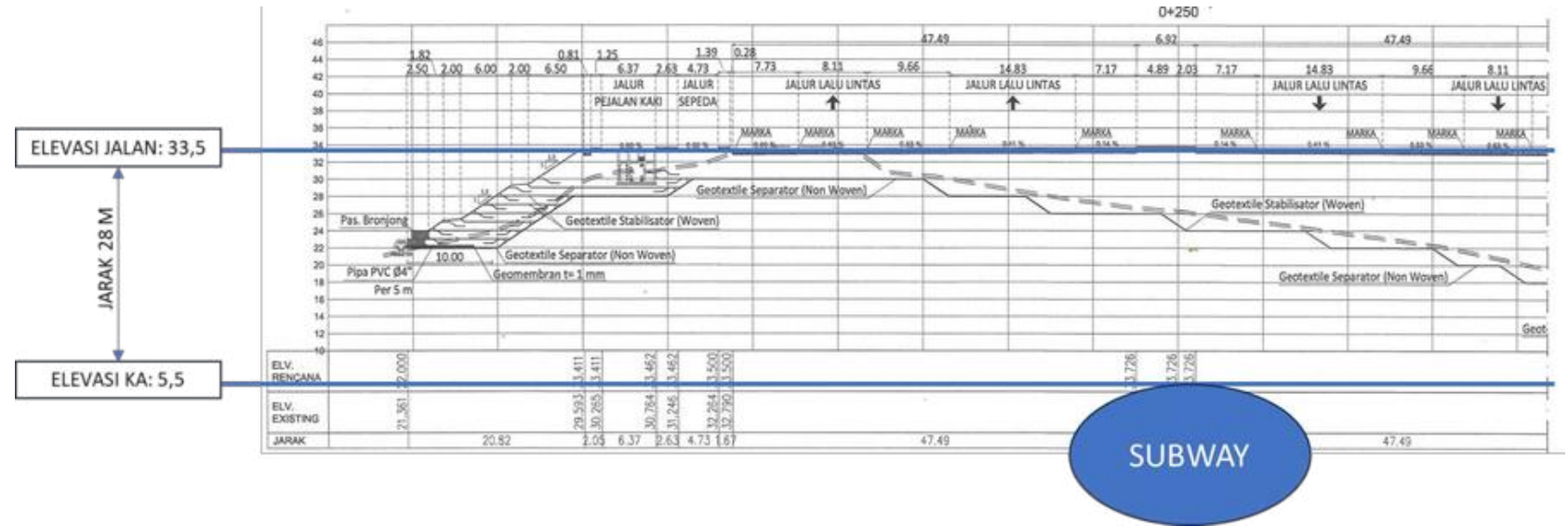
Tipikal Jalur KA Underground pada Timbunan
