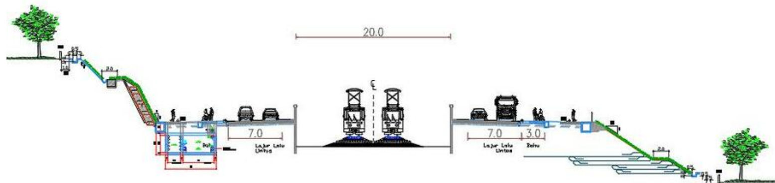
Tipikal Jalur KA At Grade /Transisi
