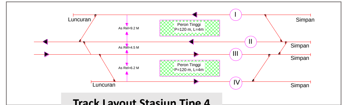
Track Layout Stasiun Tipe 4
