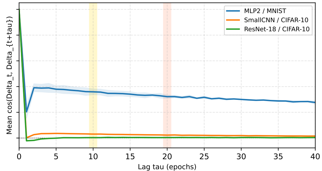
AdamW
