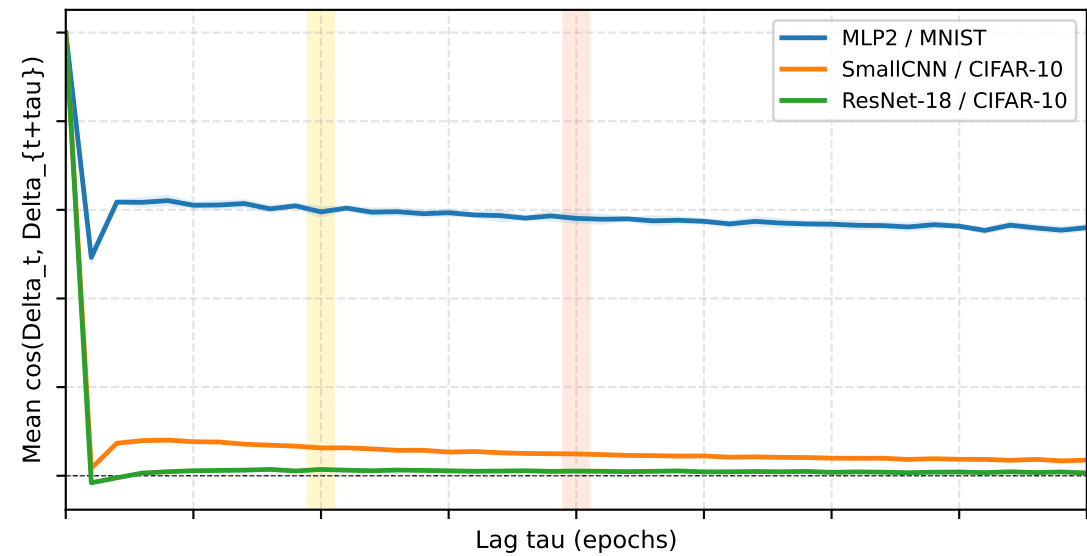
AdamW
