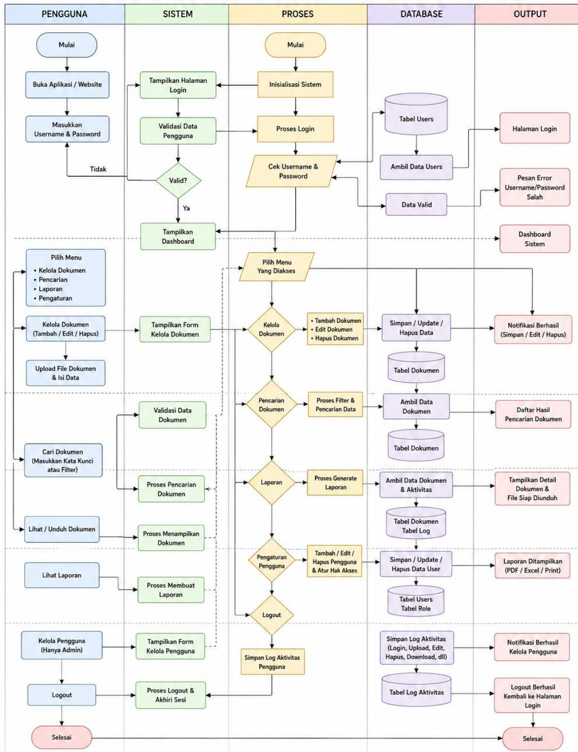
FLOWCHART SISTEM MANAJEMEN ARSIP SURAT DAN DOKUMEN DIGITAL
