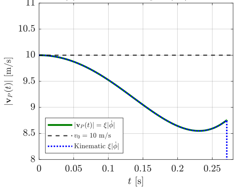
(d) Bounded Linear Speed |\mathbf{v}_P| < \infty
