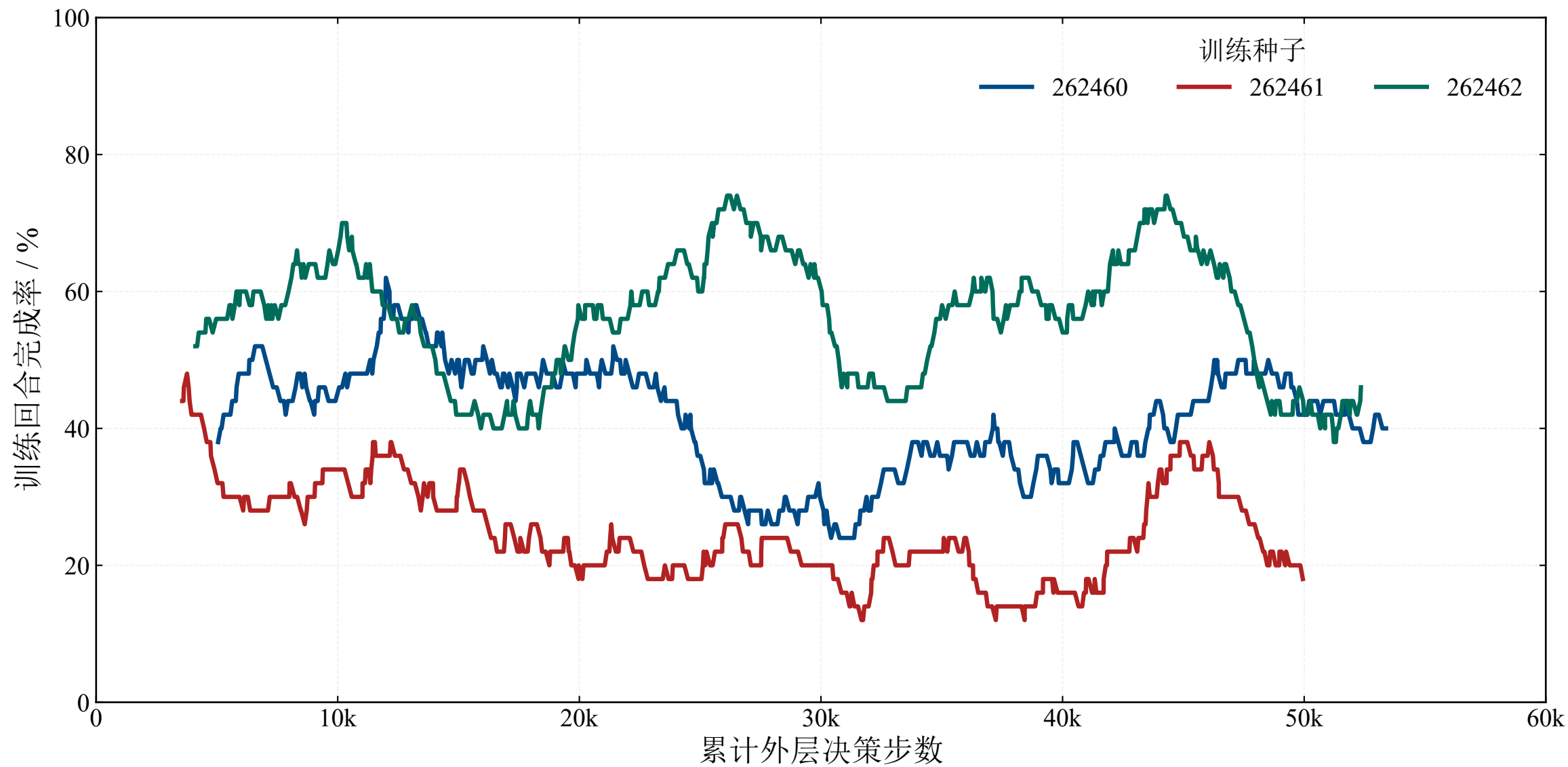
训练任务完成率
