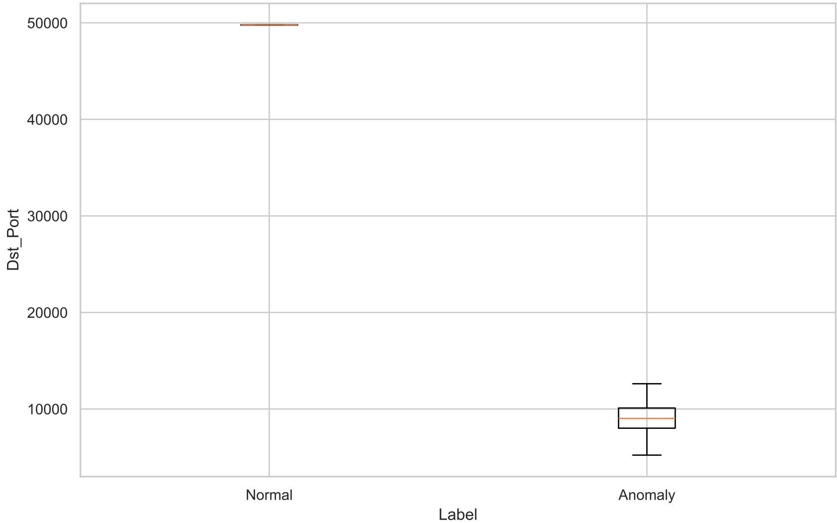
Dst_Port vs Label
