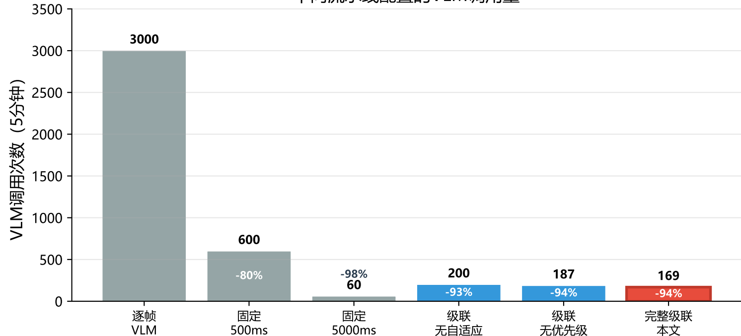
不同流水线配置的VLM调用量
