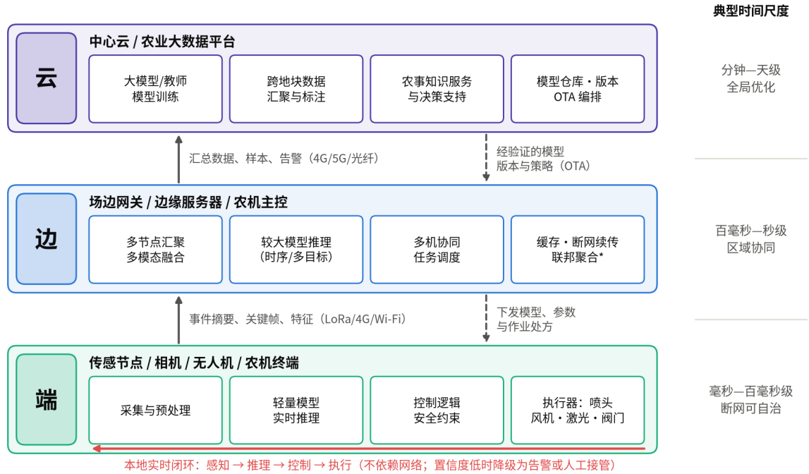
图7 智慧农业端一边一云协同总体架构
