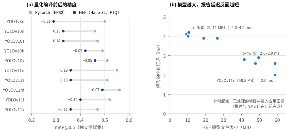
图12 Hailo 杂草研究中的量化精度损失与计时口径疑点：（a）PyTorch 与 HEF 模型的 mAP@0.5；（b）HEF 模型大小与报告延迟 自绘。数据来自文献[24]表1（作者报告）。
