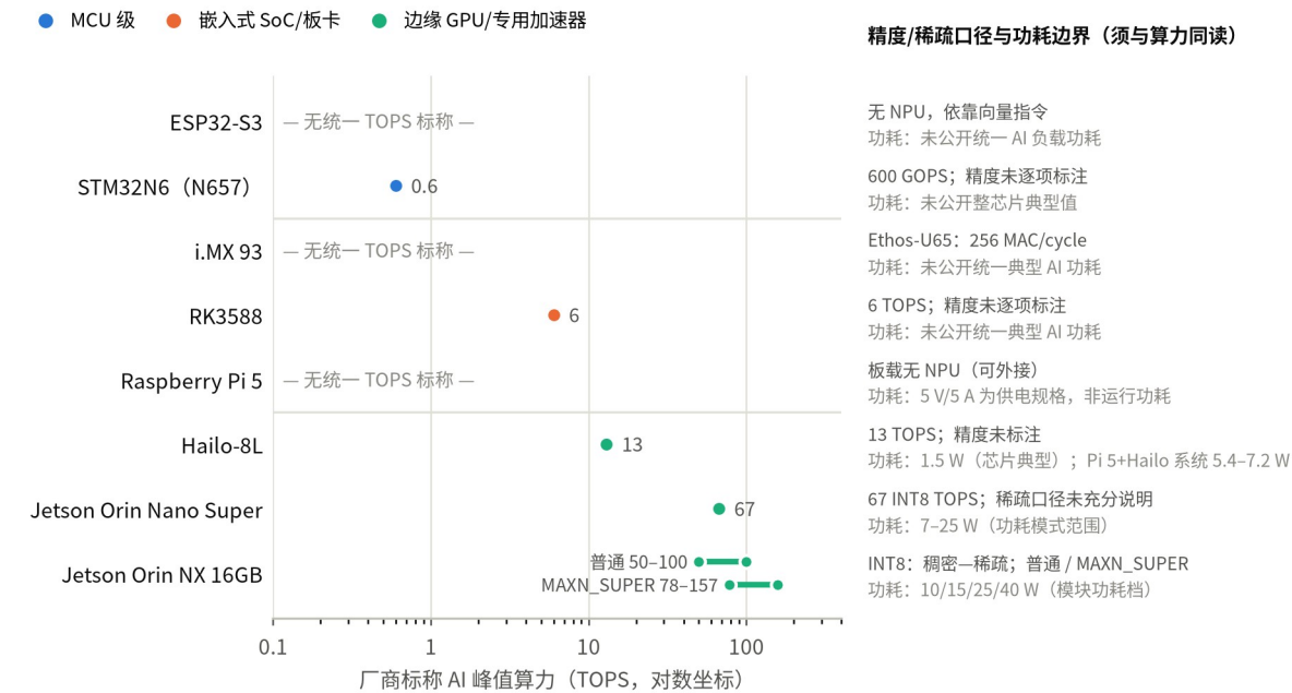
自绘。数据来自各厂商官方资料[14,15,17–21,23]与文献[24]；算力为厂商标称峰值，精度与稀疏口径不一致，不能据此直接比较能效。
