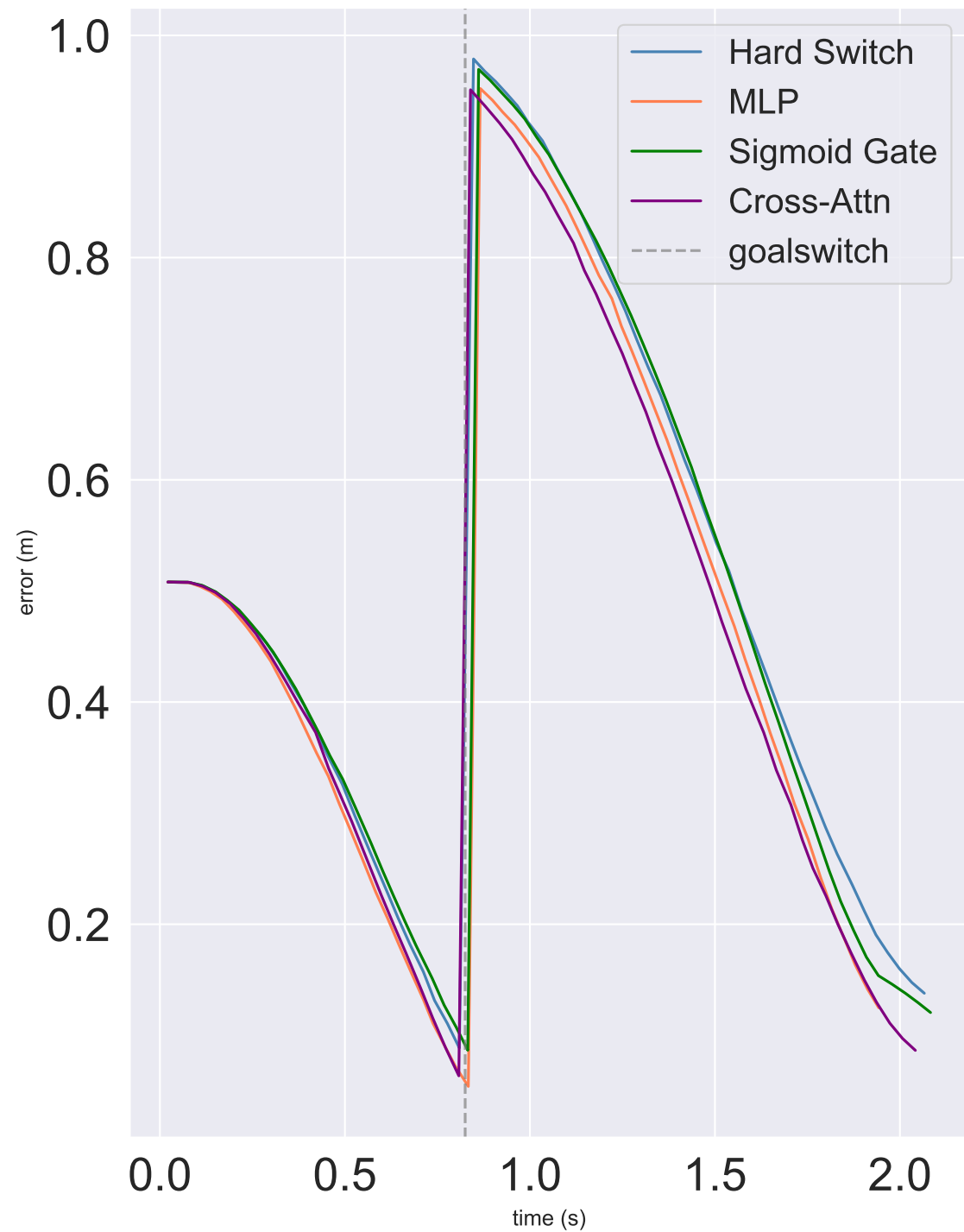
A. Position Error
