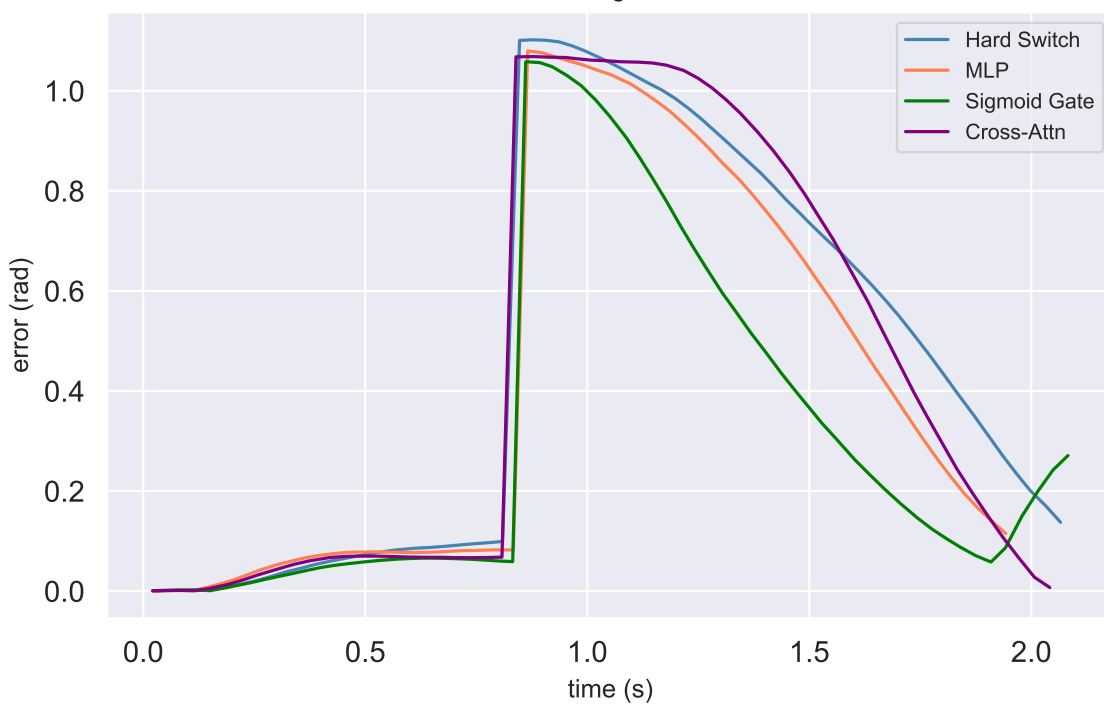
Heading Error
