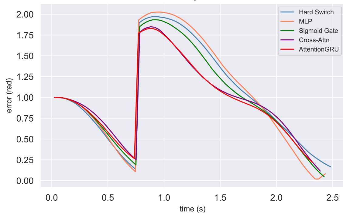
Heading Error
