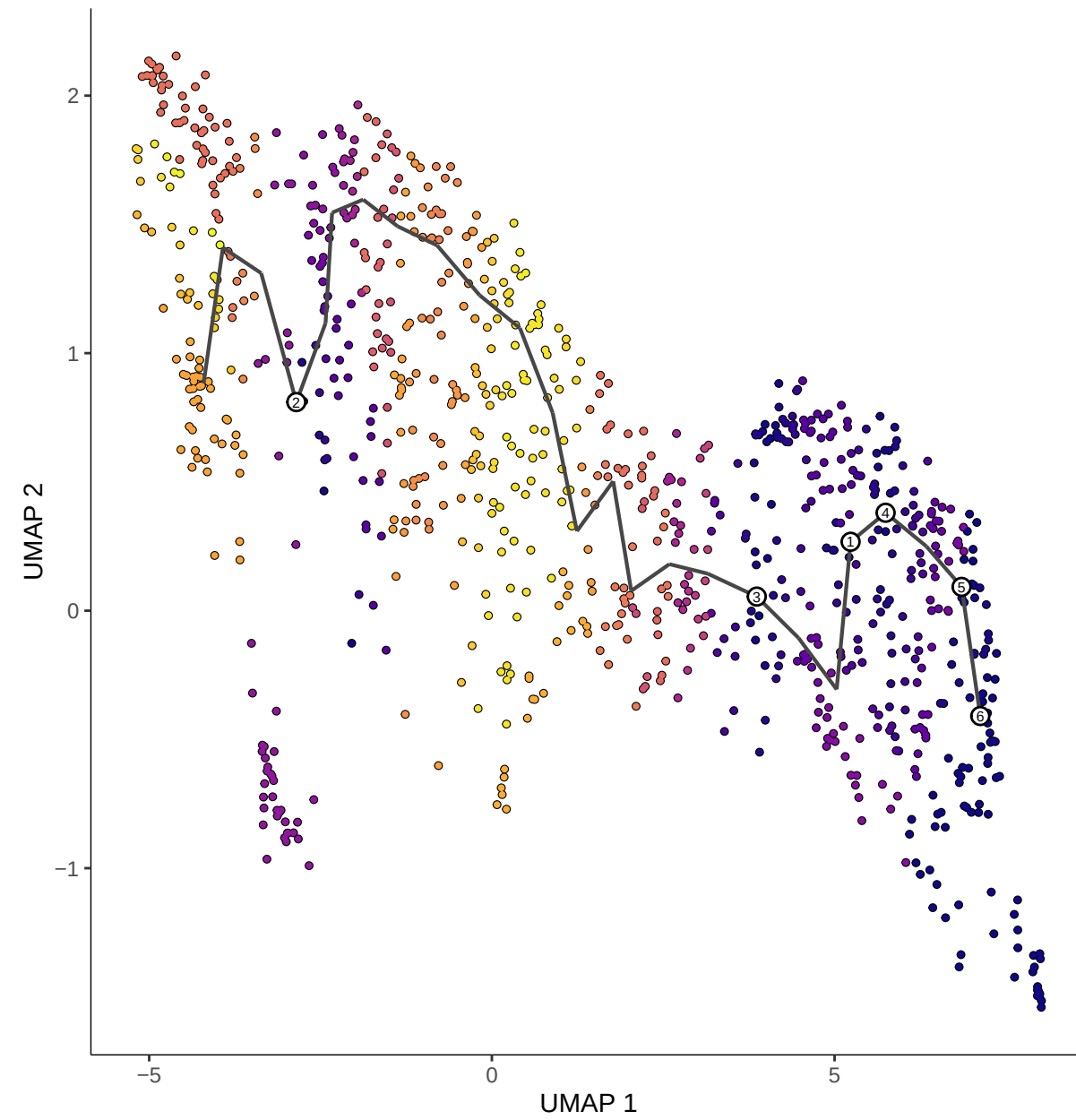
B: Pseudotime
