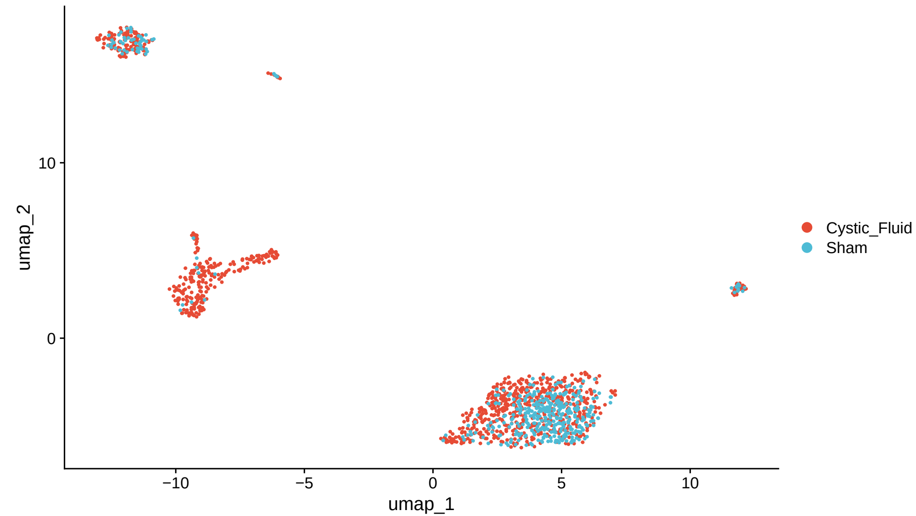
A: Microglia UMAP by Group
