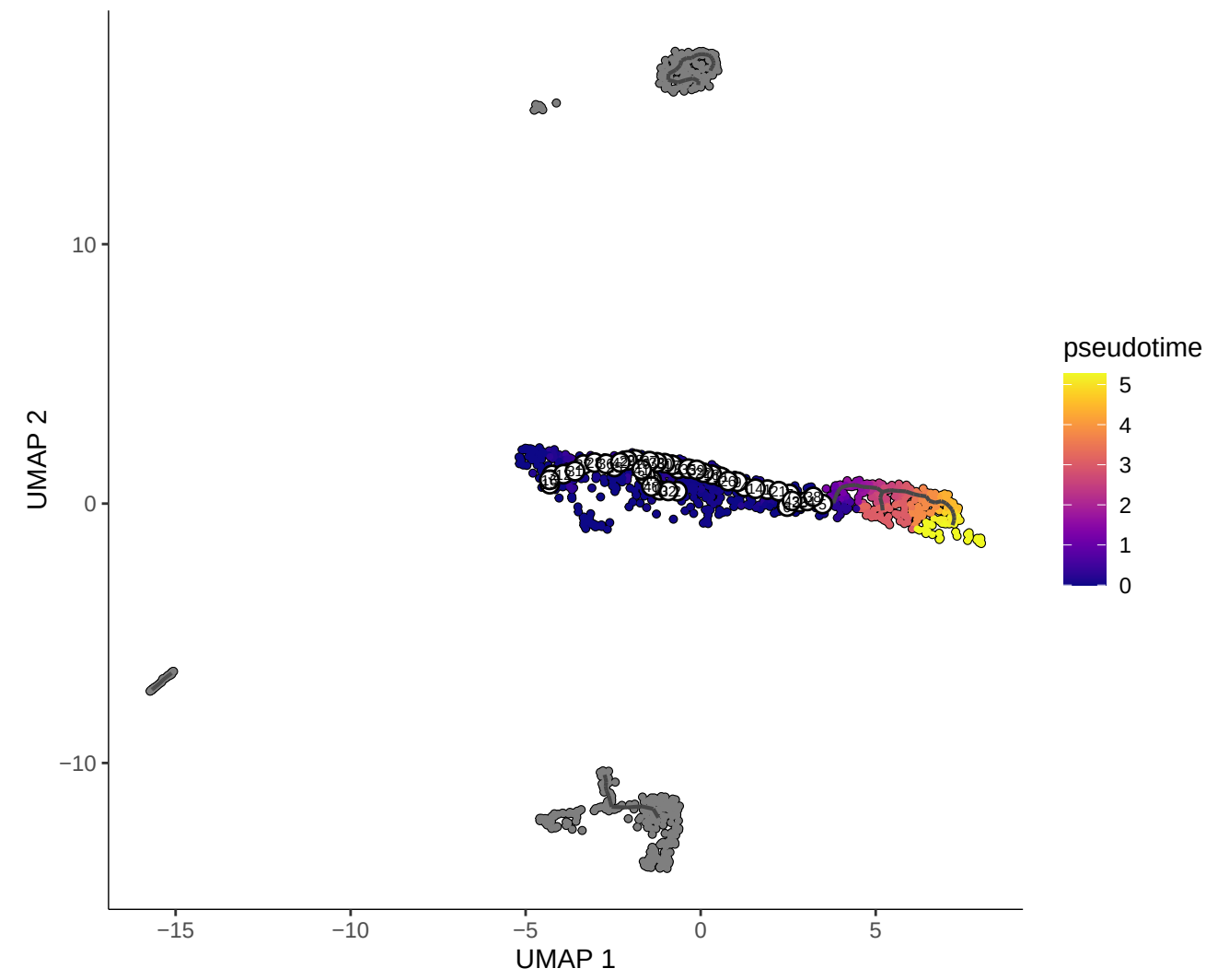
Microglia Pseudotime (Monocle3)
