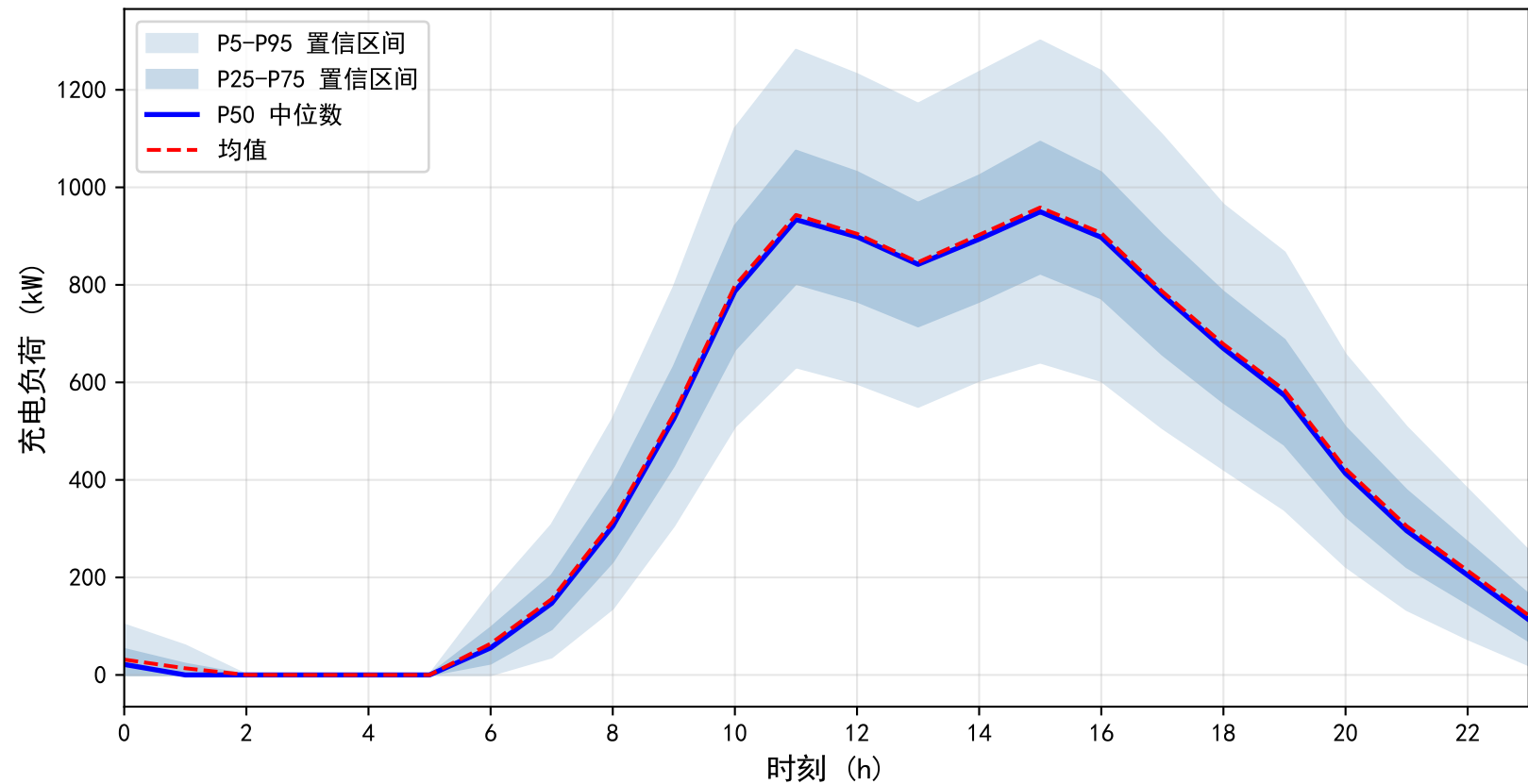
高速服务区充电负荷概率分布（工作日，中型服务区）
