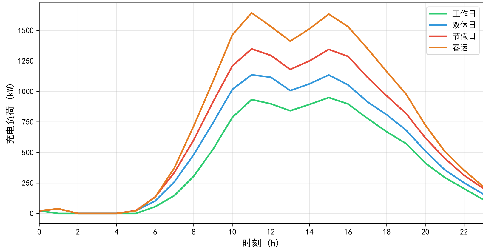
不同日类型充电负荷P50曲线对比
