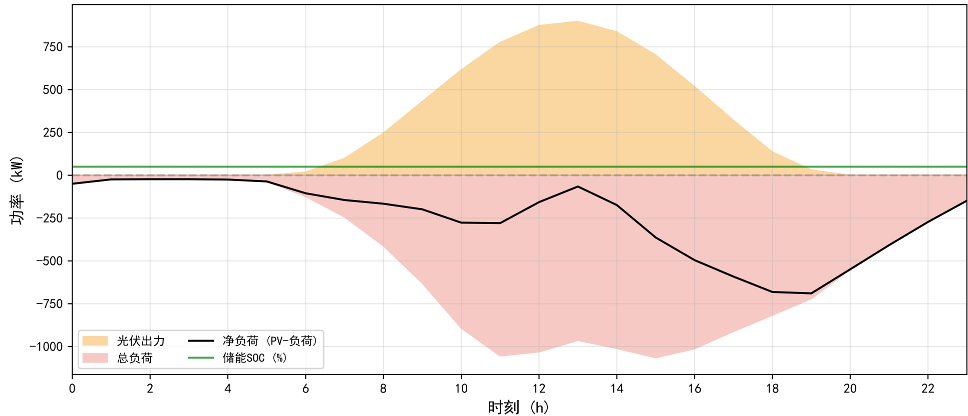
典型日功率平衡 (summer clear)
