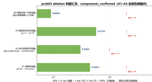
图36 硅模型的消融判定汇总
