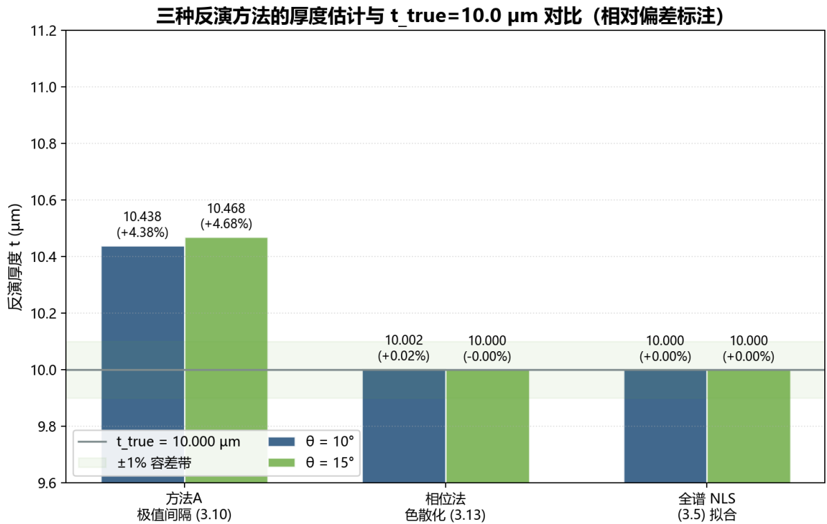
图4 三种方法的合成厚度估计
