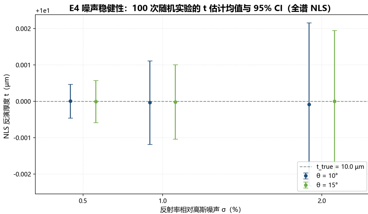
图9 不同噪声水平下的合成厚度区间
