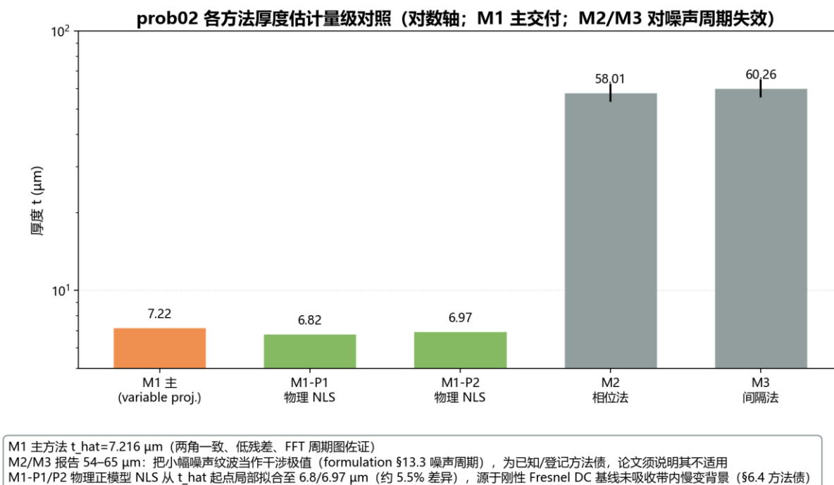
图22 碳化硅不同反演方法的厚度量级
