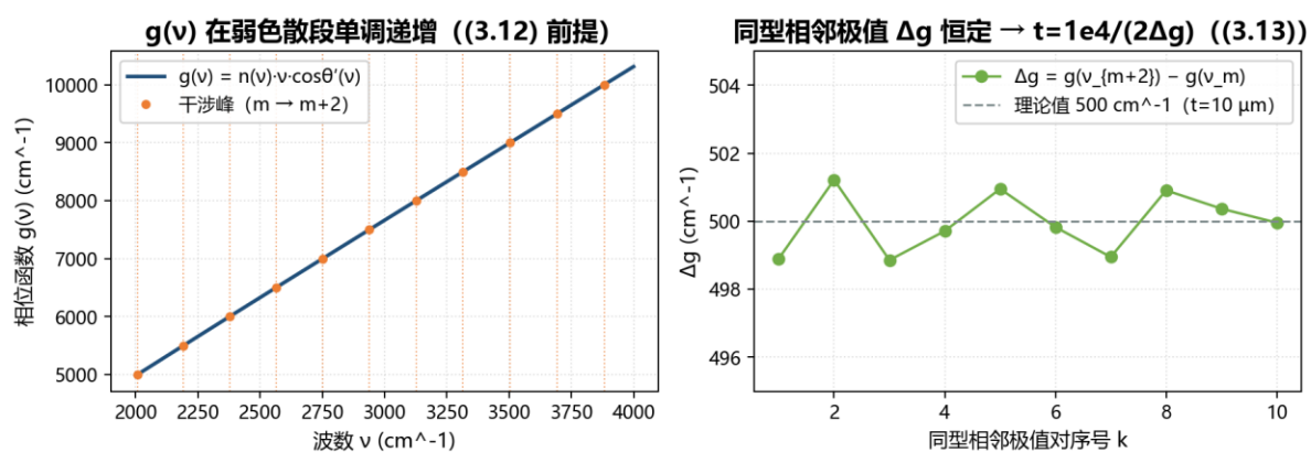
图3 相位函数与同型极值间隔
