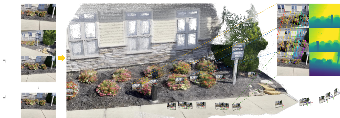
(b) VGGT
