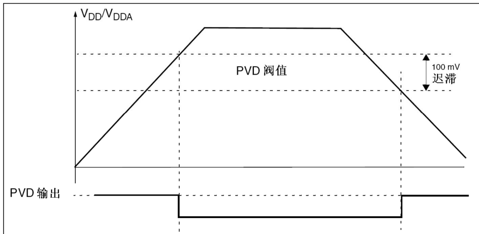
图6 PVD的门限
