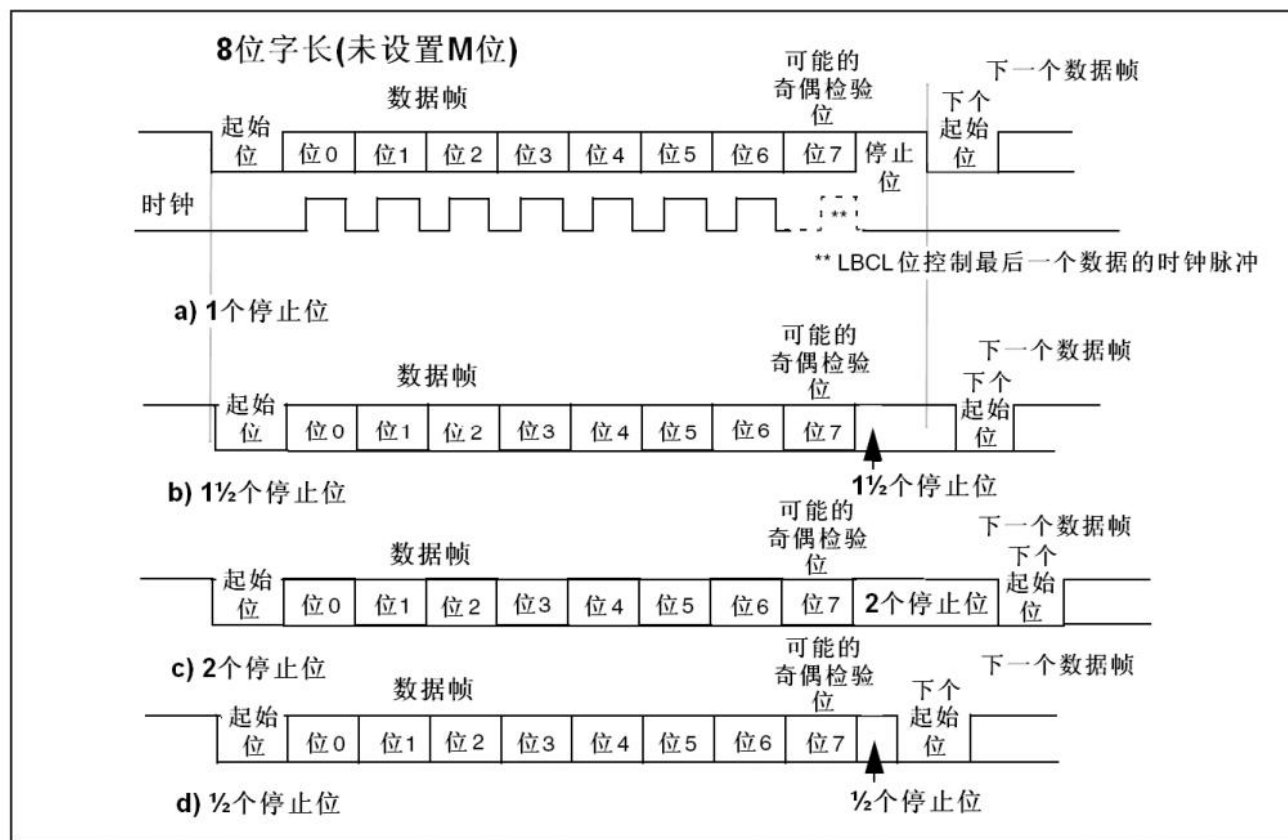
图250 配置停止位
