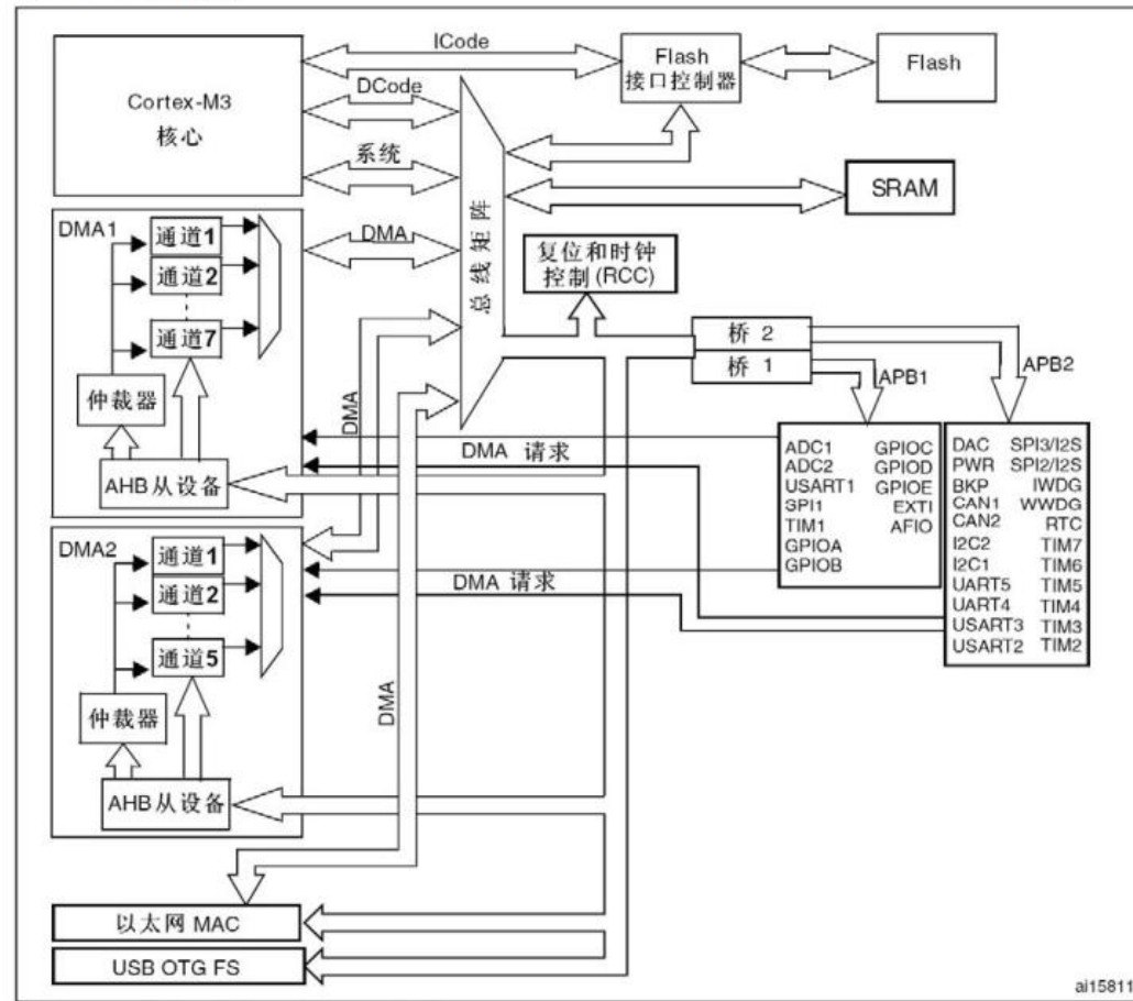
图21 DMA框图
