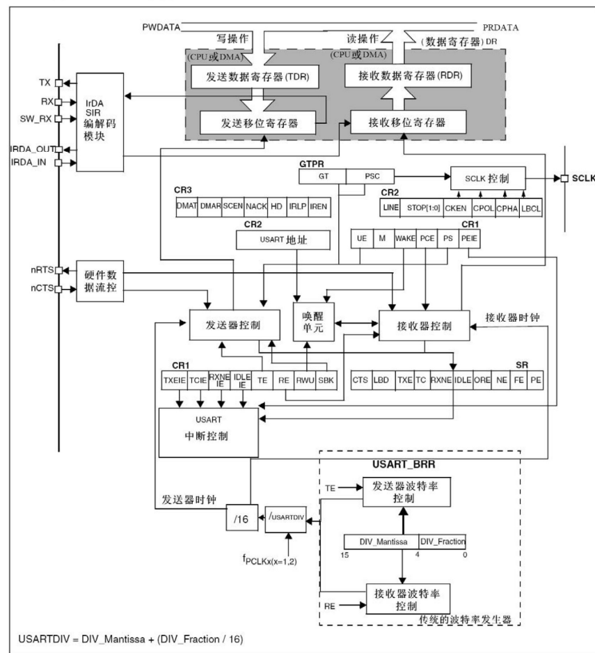
图248 USART框图
