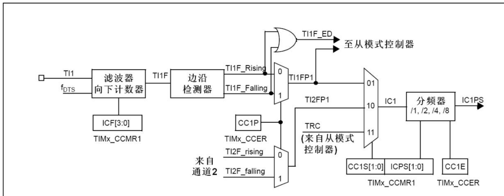
图123 捕获/比较通道(如：通道1输入部分)
