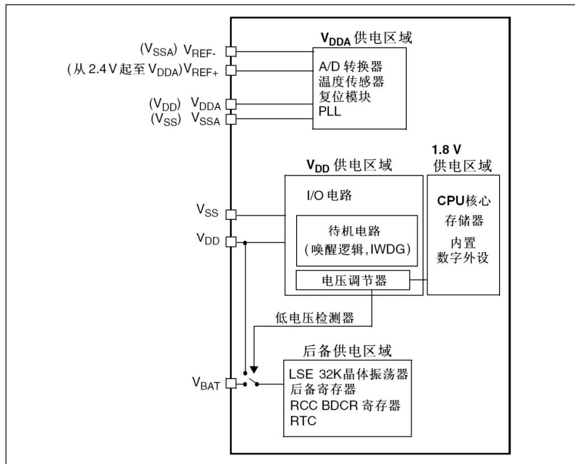
图4 电源框图
