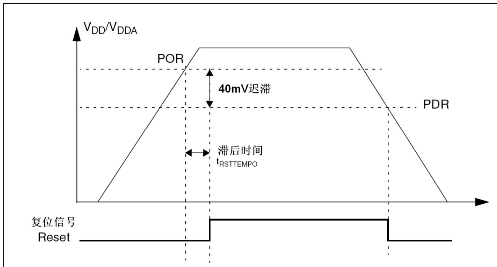
图5 上电复位和掉电复位的波形图
