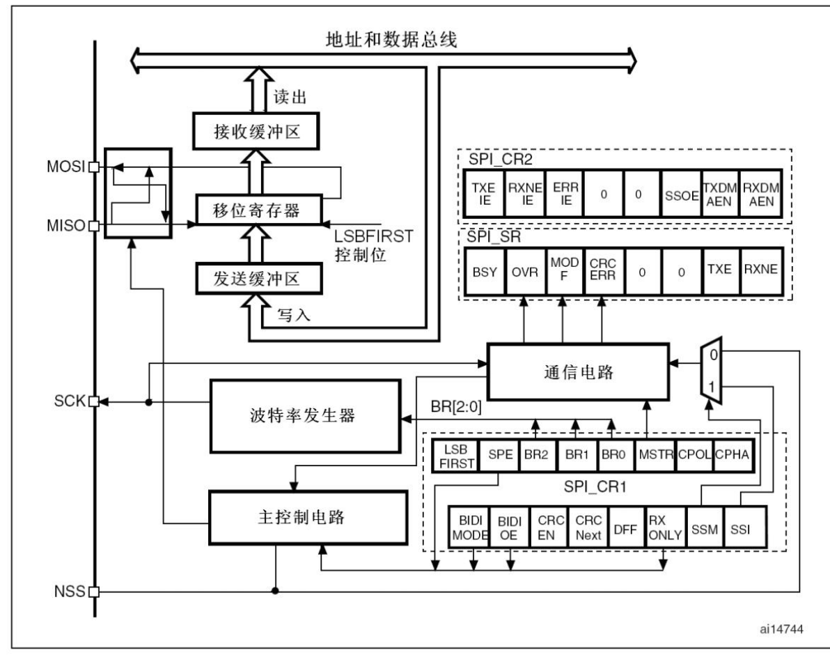
图209 SPI框图
