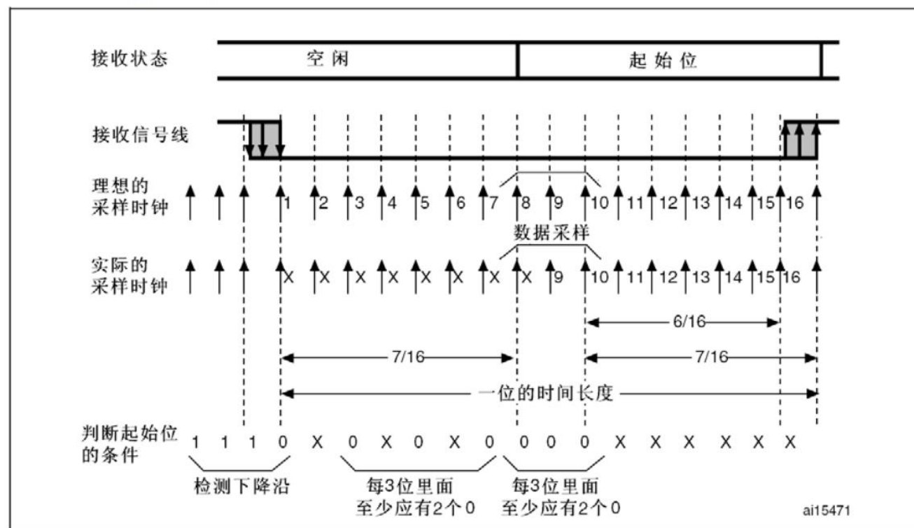
图252 起始位侦测
