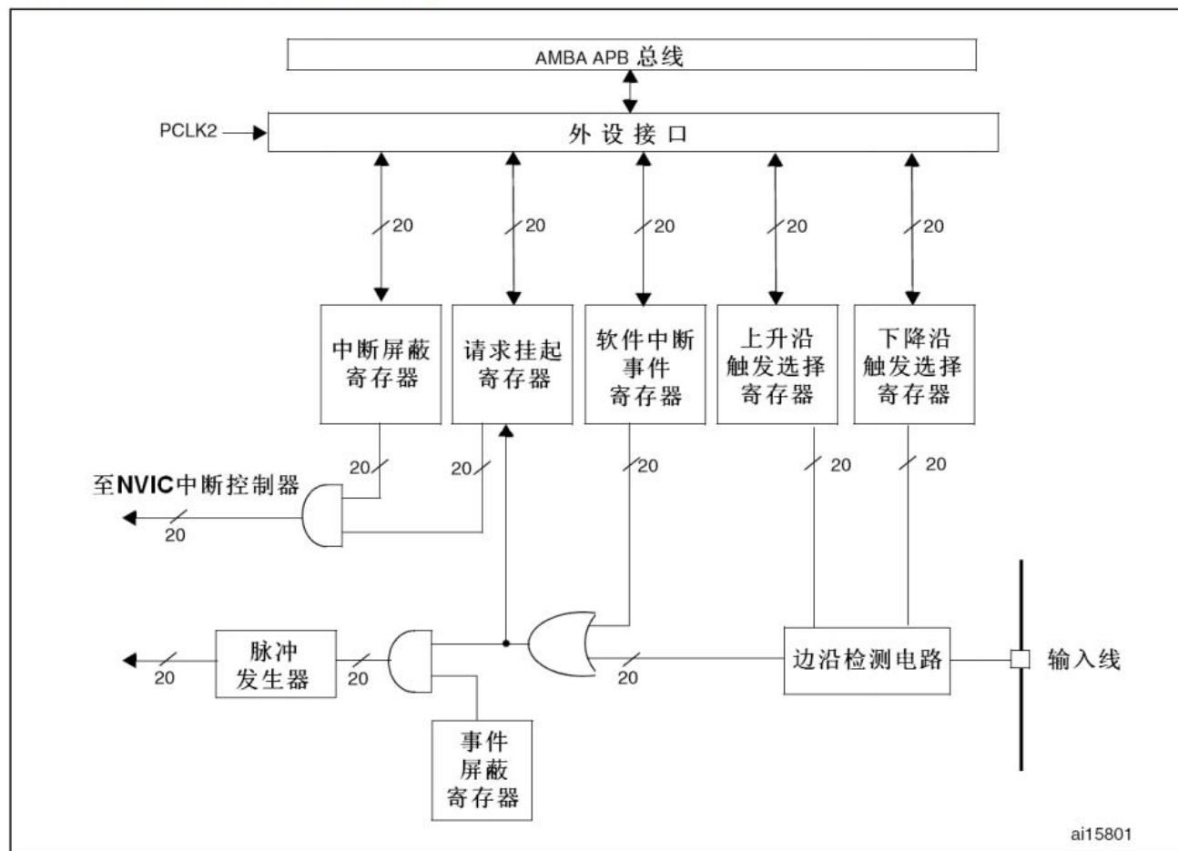
图19 外部中断/事件控制器框图
