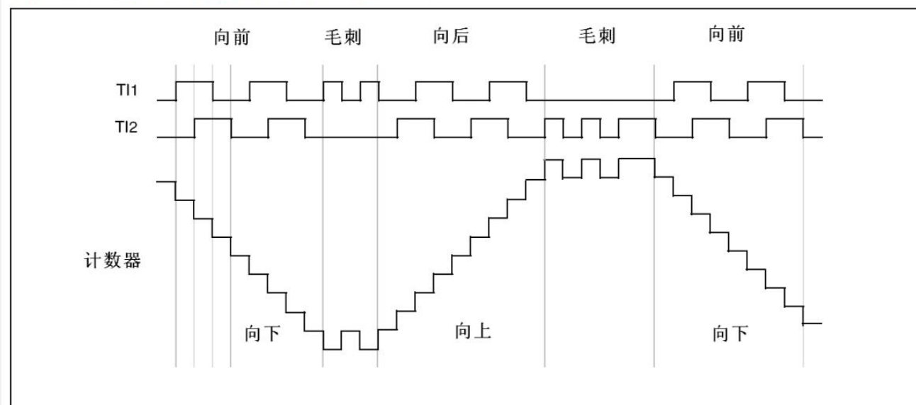
图133 IC1FP1反相的编码器接口模式实例
