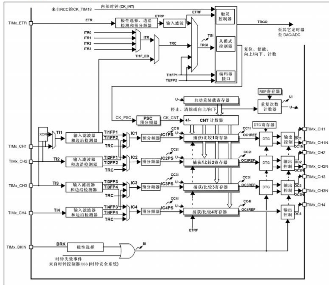
图50 高级控制定时器框图
