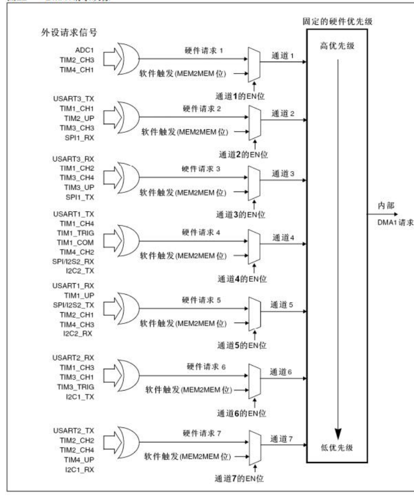
图22 DMA1请求映像
