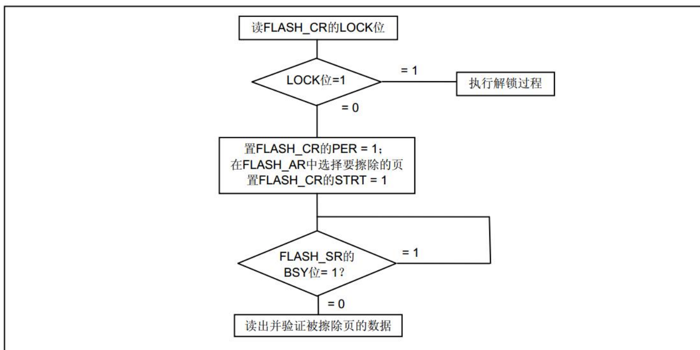
图二 闪存页擦除过程
