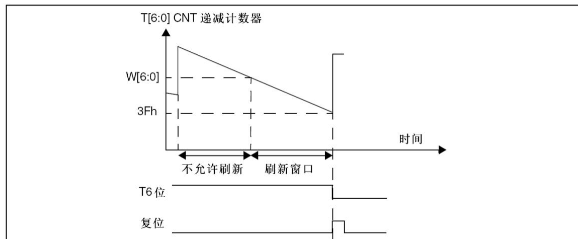
图159 窗口看门狗时序图
