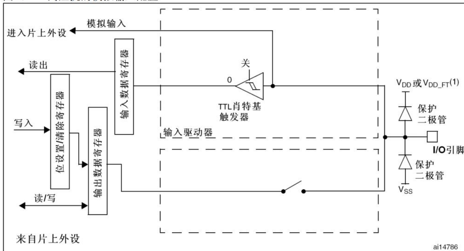
图18 高阻抗的模拟输入配置
