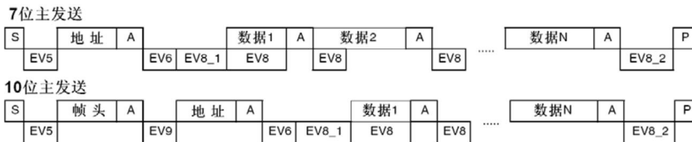
图245 主发送器传送序列图
