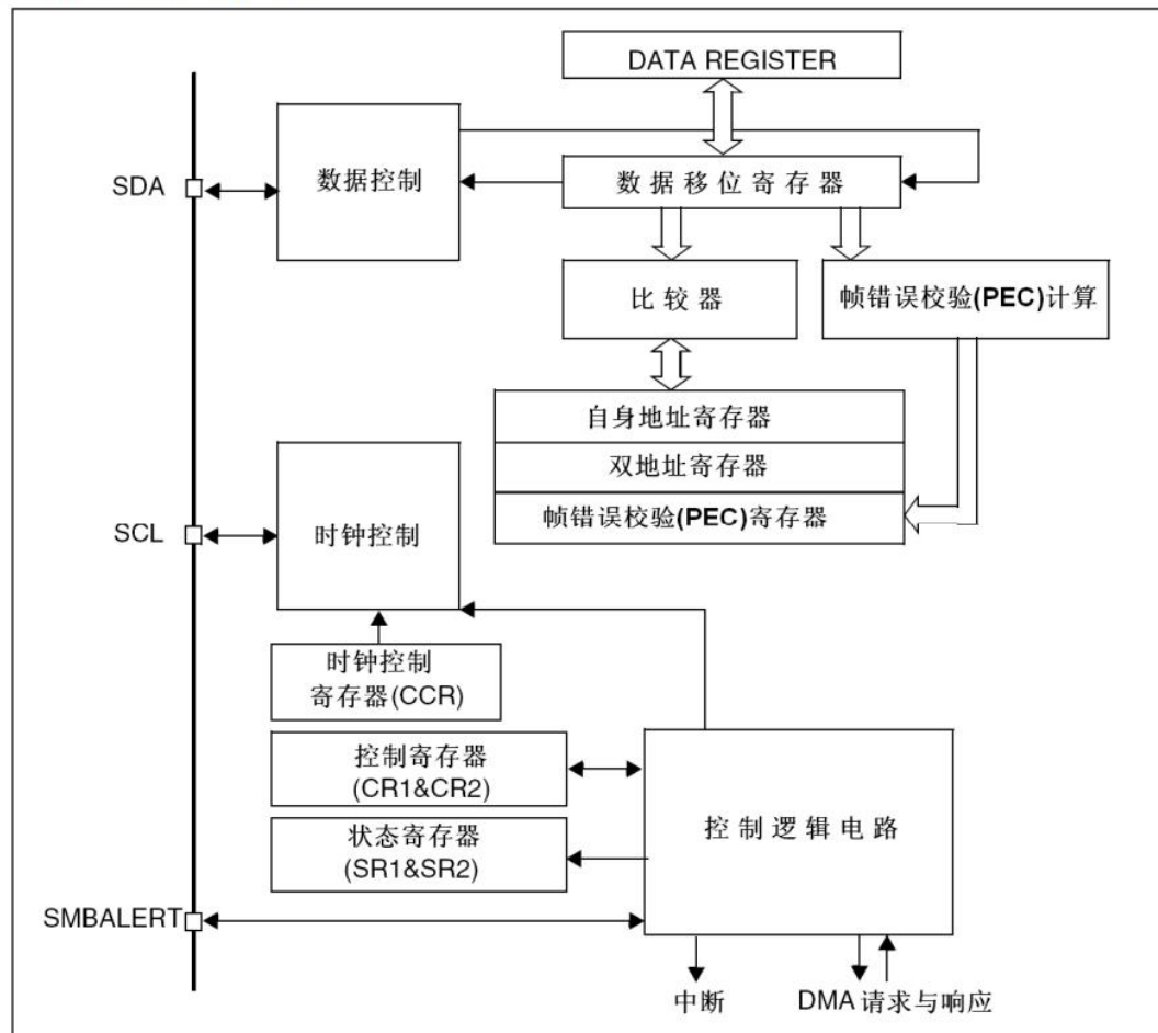
图242 I 2 C的功能框图
