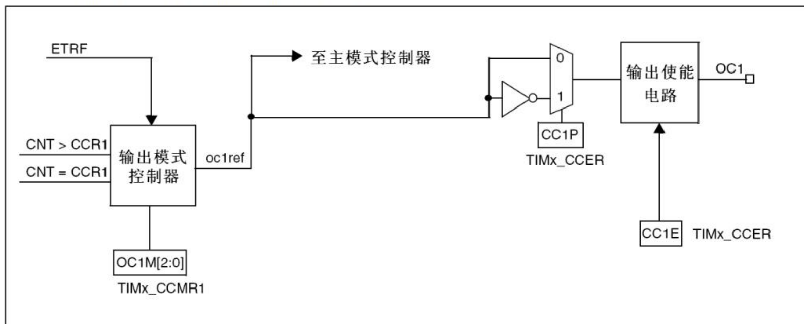
图125 捕获/比较通道的输出部分(通道1)
