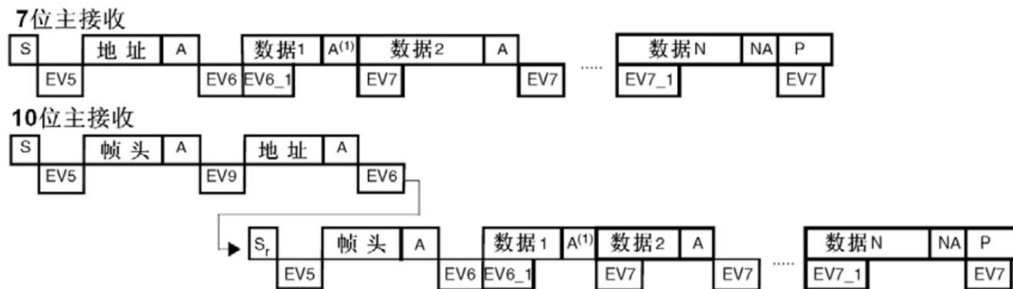
图246 主接收器传送序列图
