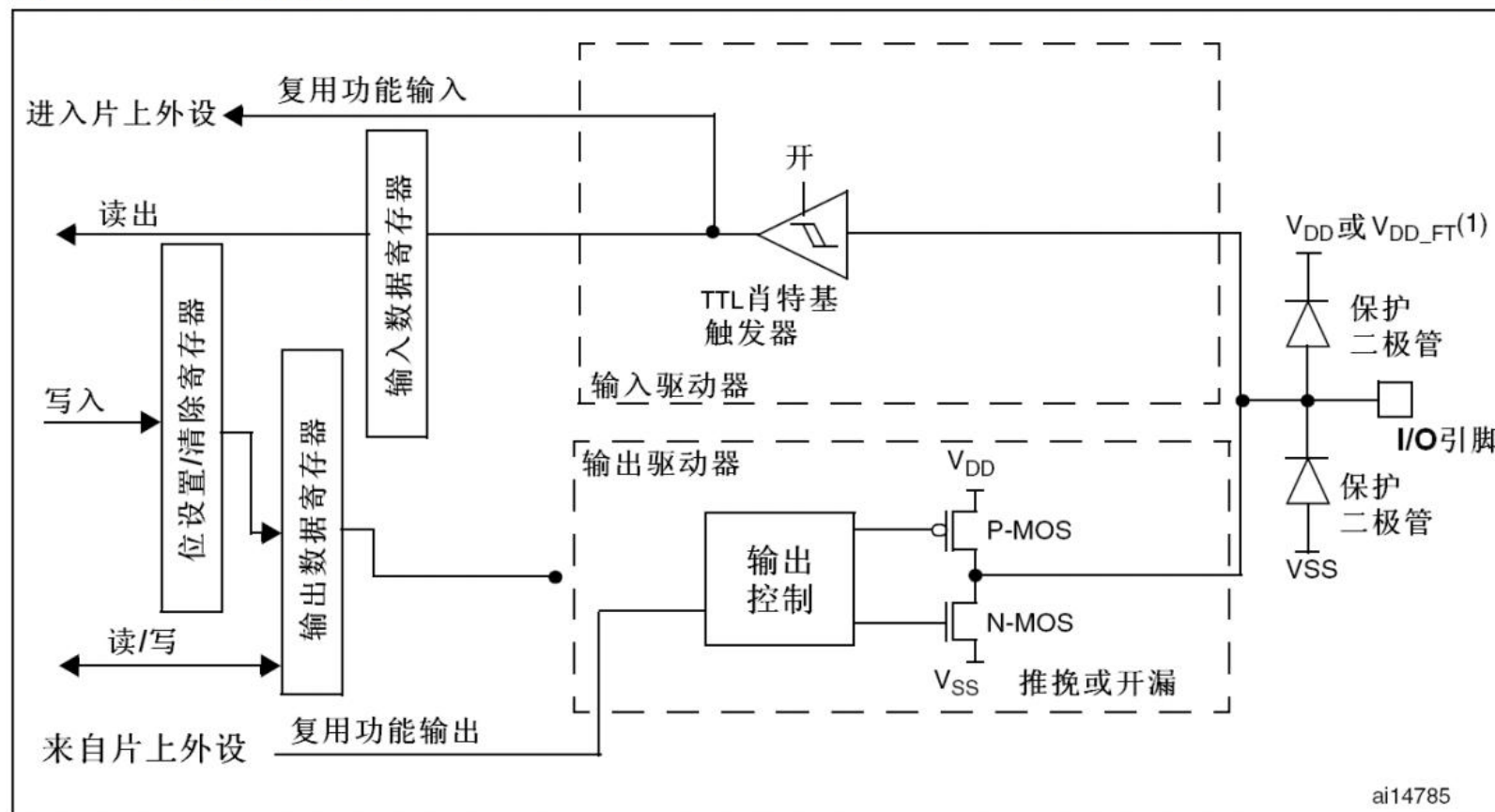
图17 复用功能配置
