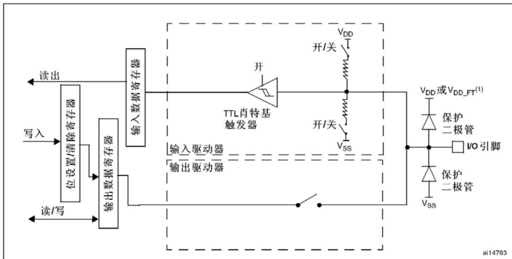
图15 输入浮空/上拉/下拉配置
