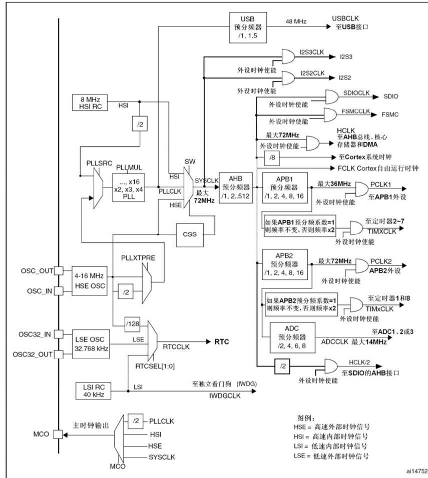
图8 时钟树
