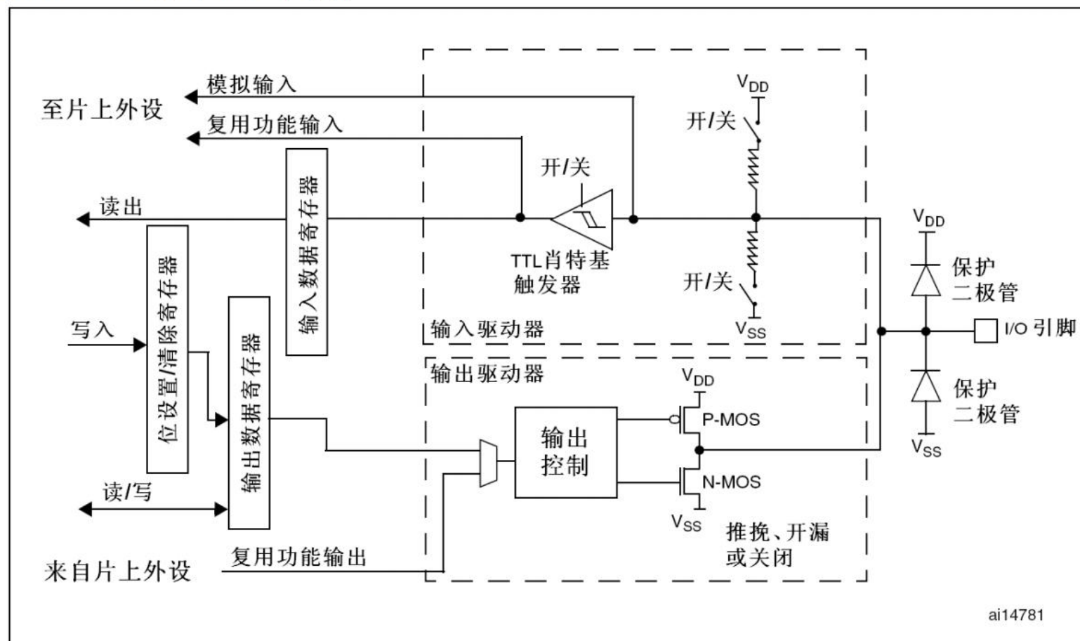
图13 I/O端口位的基本结构
