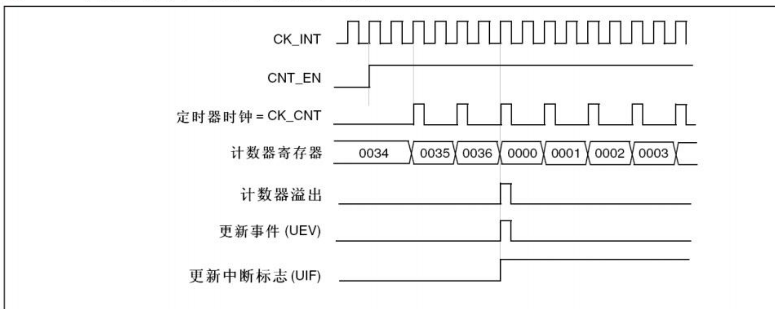
图102 计数器时序图，内部时钟分频因子为2
