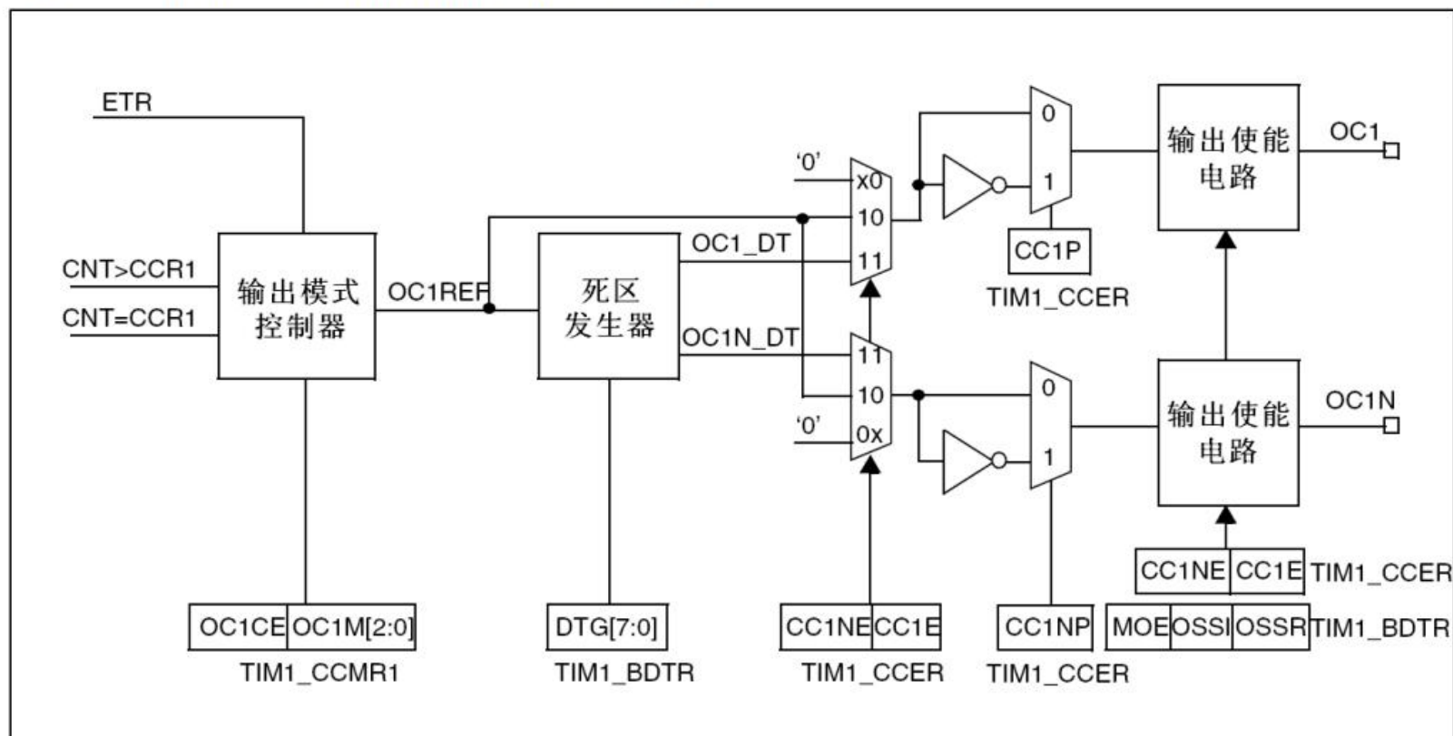
图78 捕获/比较通道的输出部分(通道1至3)
