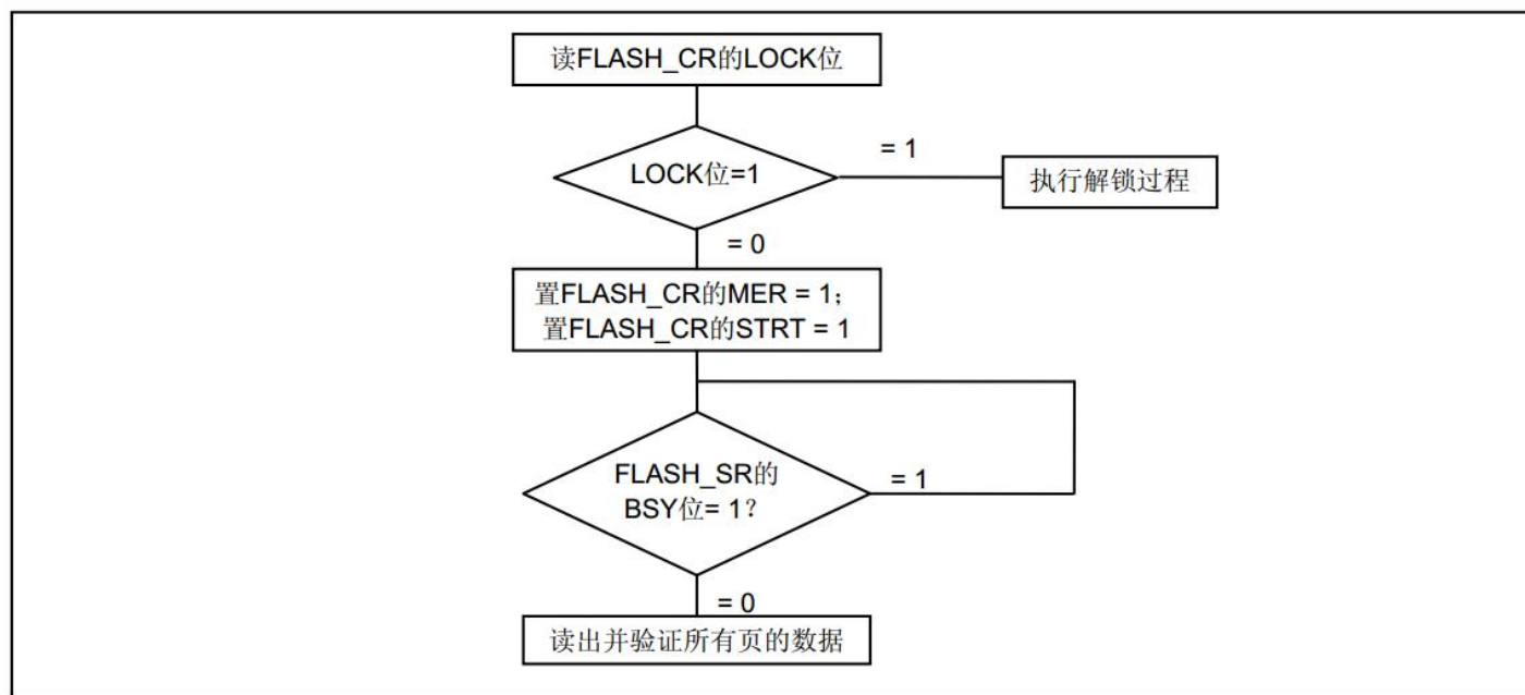
图三 闪存全擦除过程
