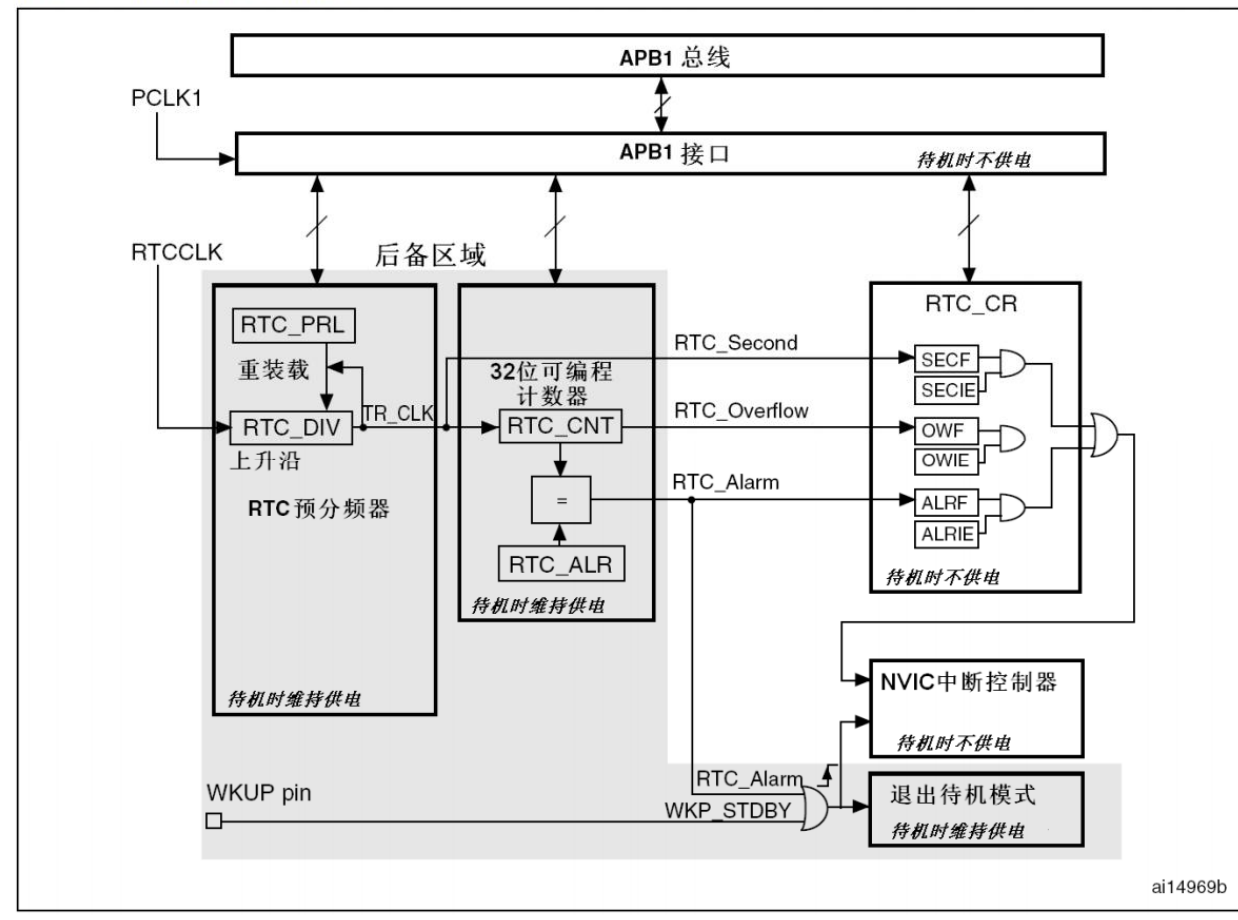
图154 简化的RTC框图
