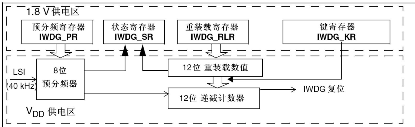
图157 独立看门狗框图
