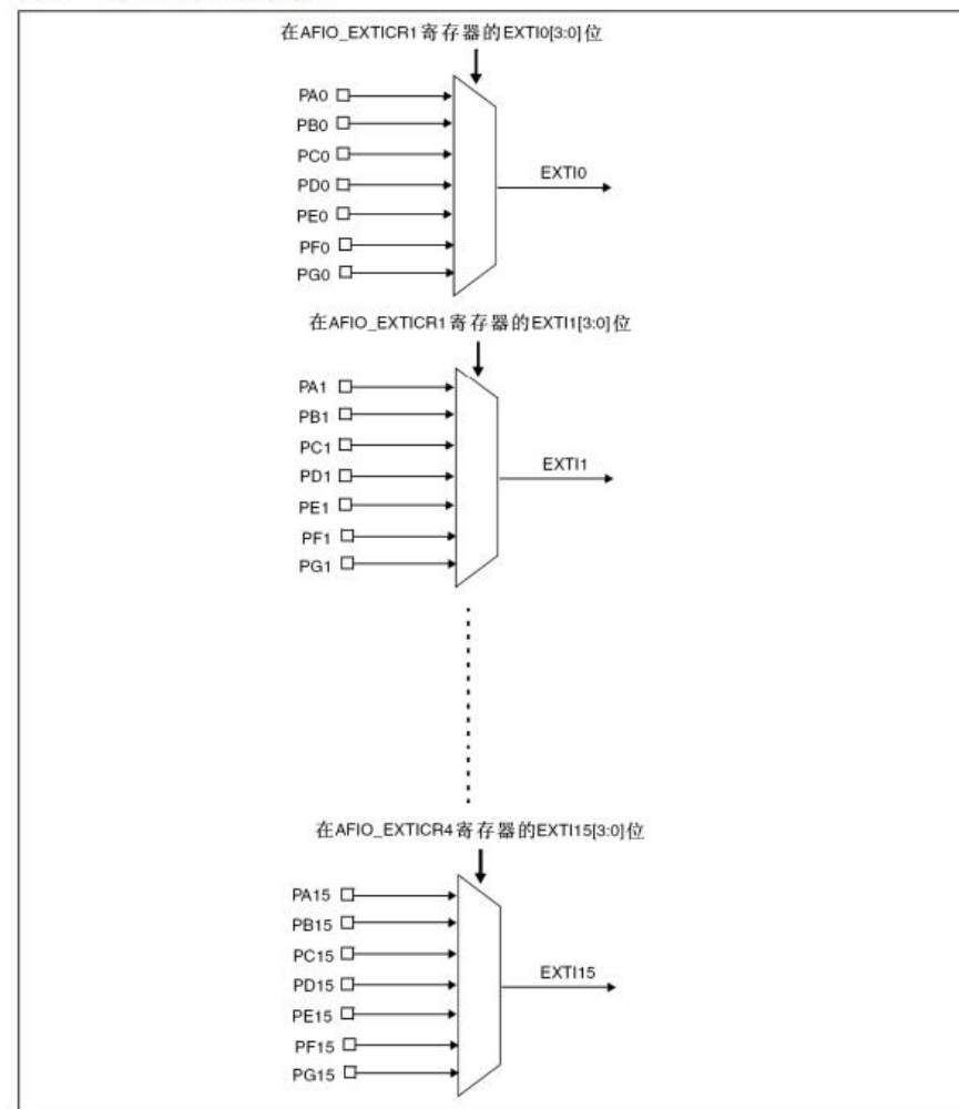
图20 外部中断通用I/O映像
