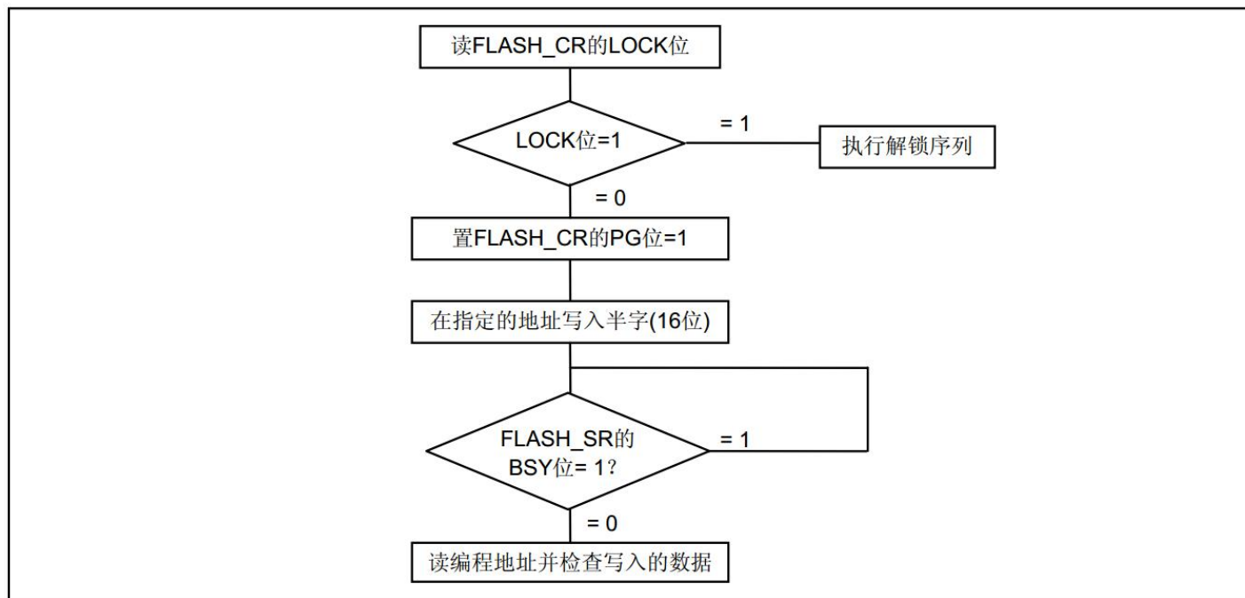
图一 编程过程
