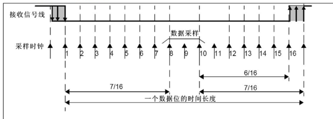
图253 检测噪声的数据采样
