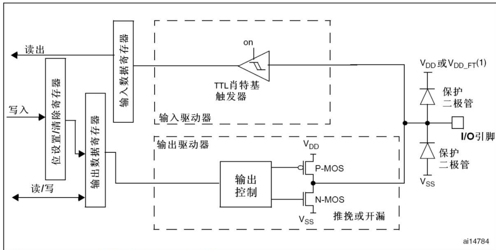
图16 输出配置
