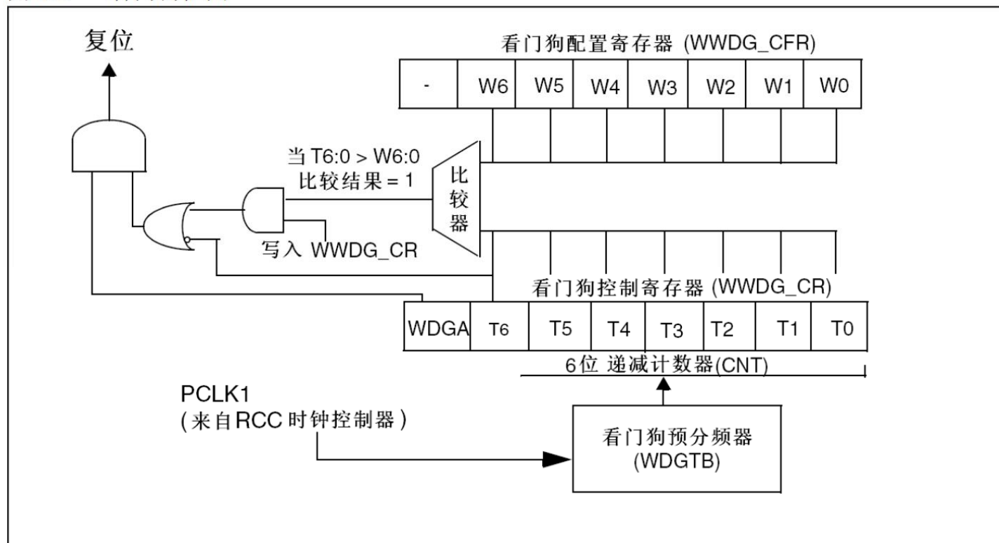
图158 看门狗框图
