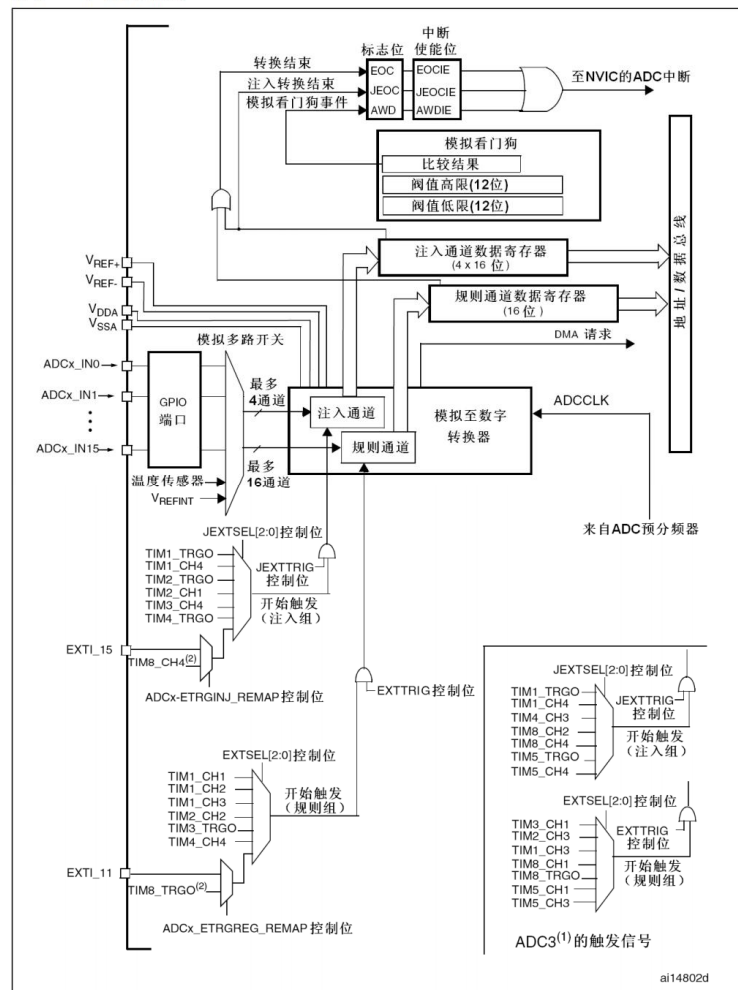
图24 单个ADC框图
