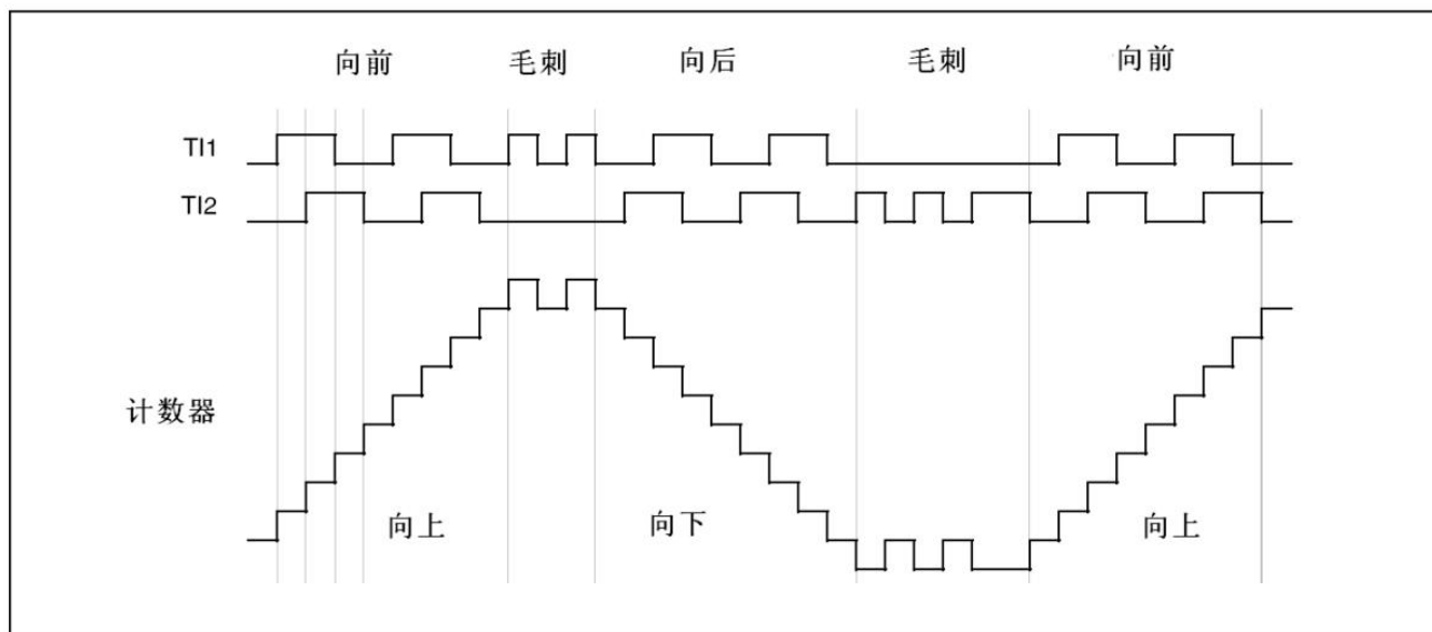
图132 编码器模式下的计数器操作实例
