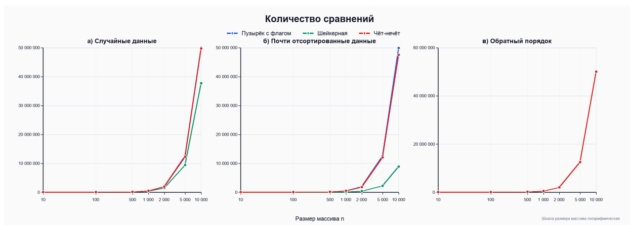
Рисунок 6 — Количество сравнений элементов при различных типах исходных данных
