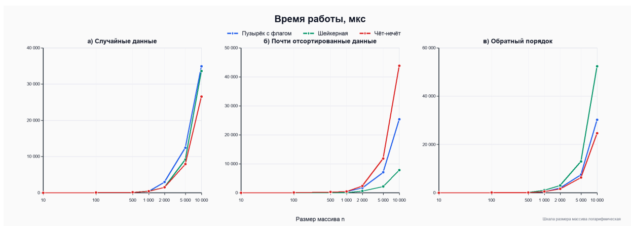
Рисунок 5 — Время работы алгоритмов при различных типах исходных данных
