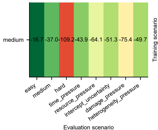
maskable ppo
