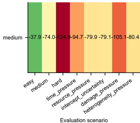
maskable ppo
