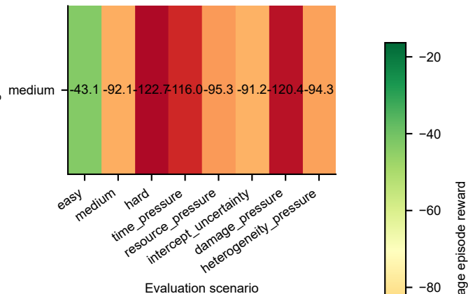
ppo
