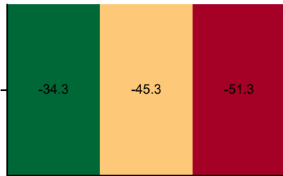
maskable ppo
