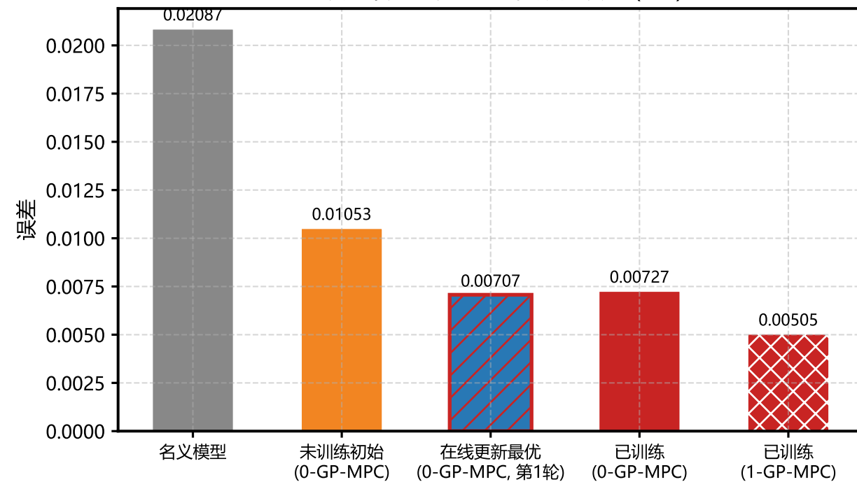
驱动力不足工况 — 均值航向误差 (rad)
