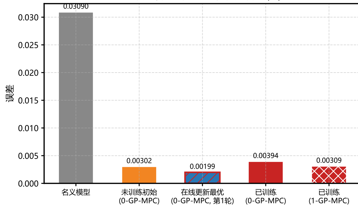
驱动力不足工况 — 均值横向误差 (m)
