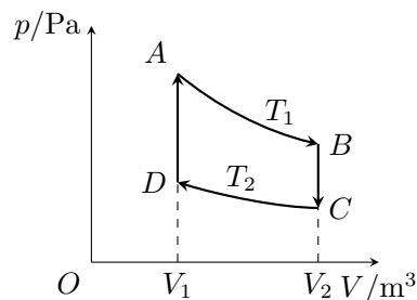
图 1: 斯特林循环
