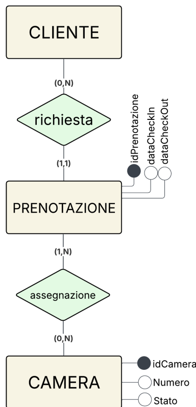
Figura 2.2: Schema E/R con associazione Prenotazione-Camera multi-a-molti
