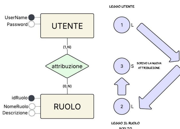
Figura 3.10: Schema di navigazione — Assegna ruolo a utente
