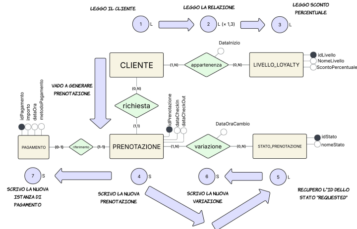
Figura 3.2: Schema di navigazione — Crea prenotazione
