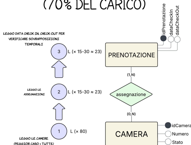
Figura 3.8: Schema di navigazione — Consulta disponibilità camere
