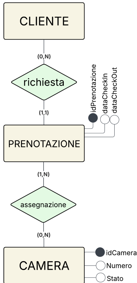
Figura 2.2: Schema E/R con associazione Prenotazione-Camera multi-a-molti
