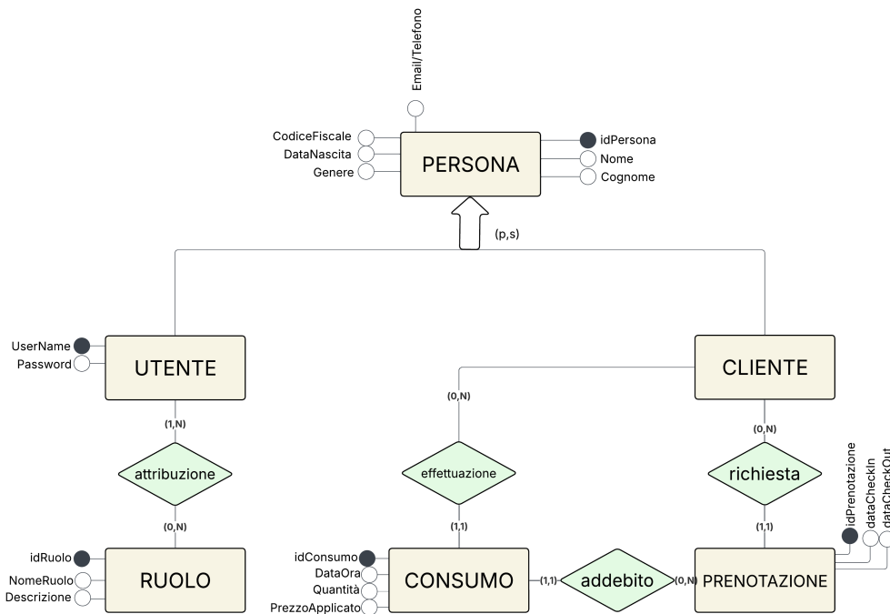
Figura 2.1: Schema E/R con le principali entità per mostrare la generalizzazione inserita nel progetto
