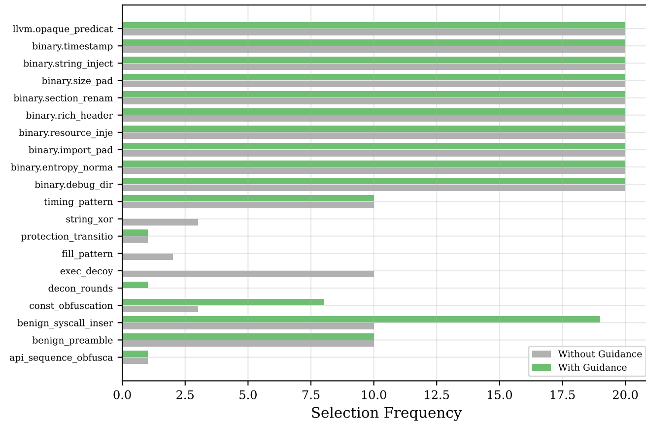
Token
