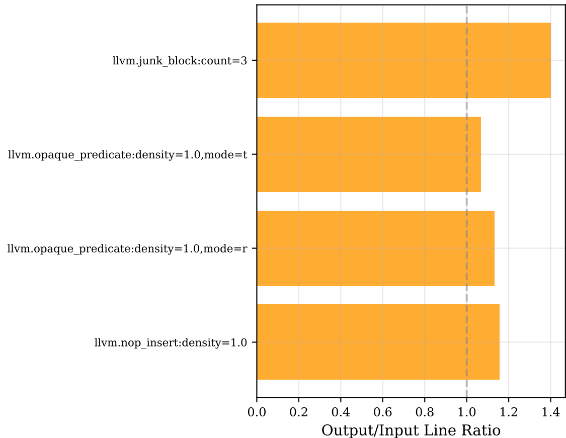
I3: IR Line Bloat
