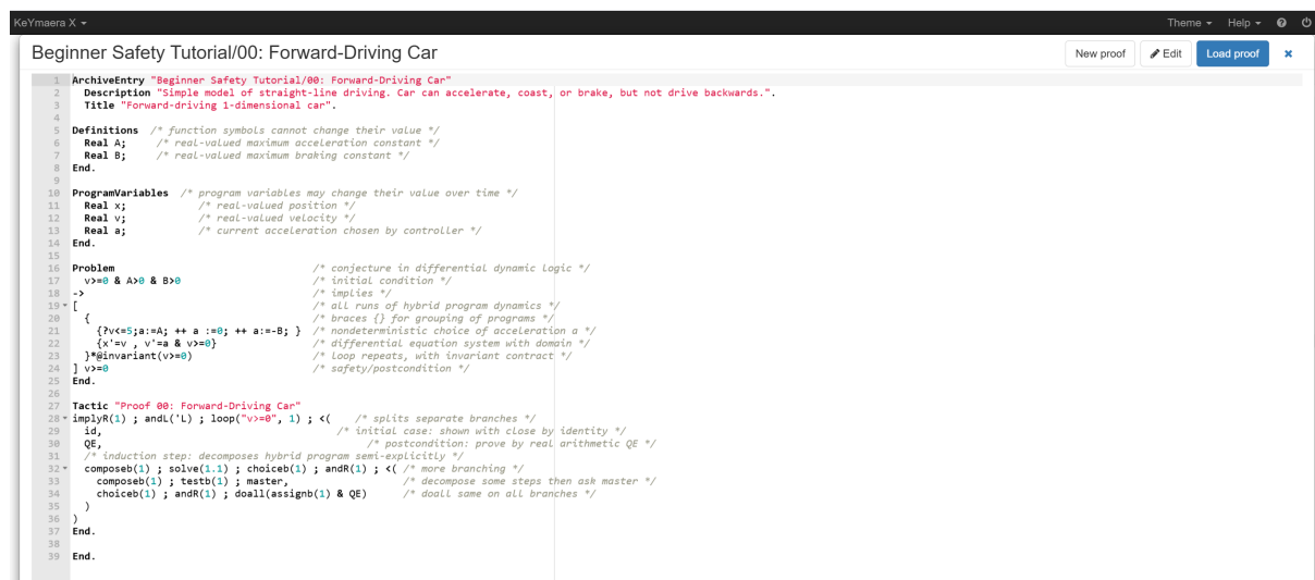
图 2.13: KeYmaera X 模型编辑 [KeYmaera X 模型编辑]
