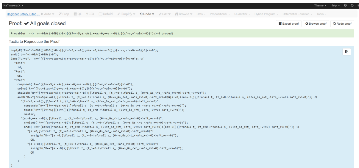
图 2.14: KeYmaera X 证明界面截图
