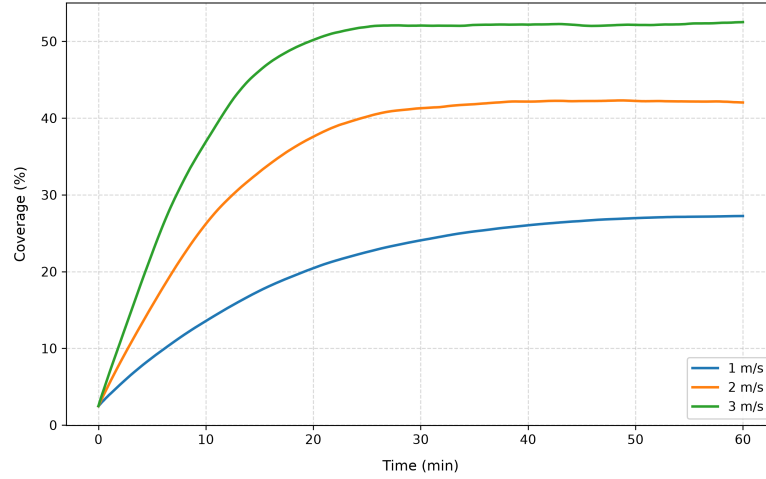
Figura 4.12: Confronto dell'evoluzione temporale della copertura al variare della velocità nominale degli agenti.
