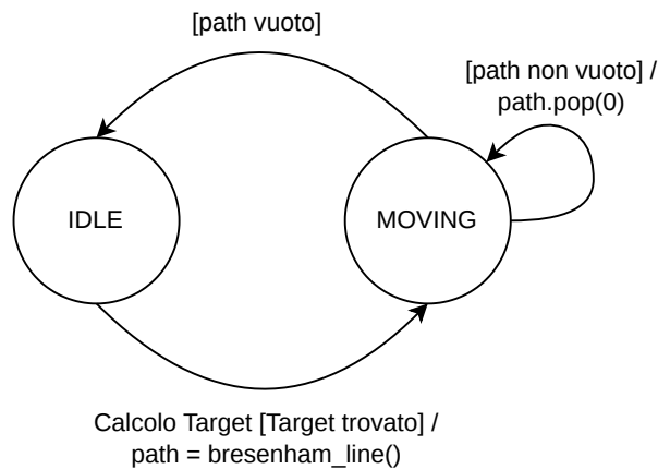
Figura 3.1: Diagramma degli stati dell'agente (Modello di Mealy).
