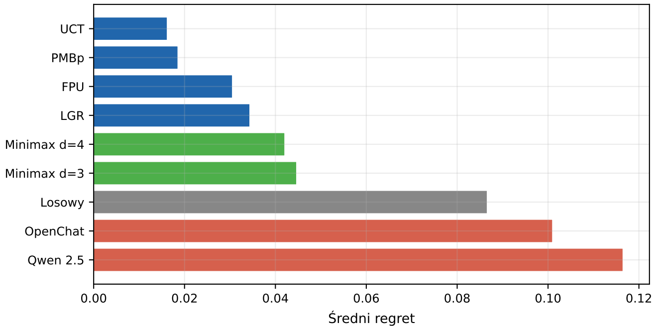
Średnia strata jakości ruchu względem wyroczni
