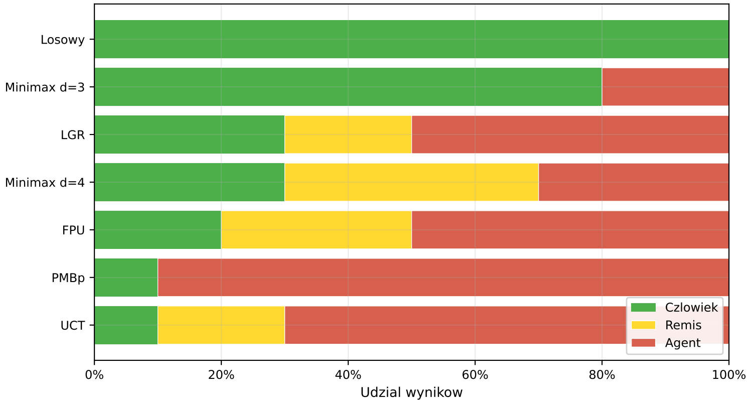
Wyniki testów człowiek-komputer (5 uczestników, 2 partie na parę)
