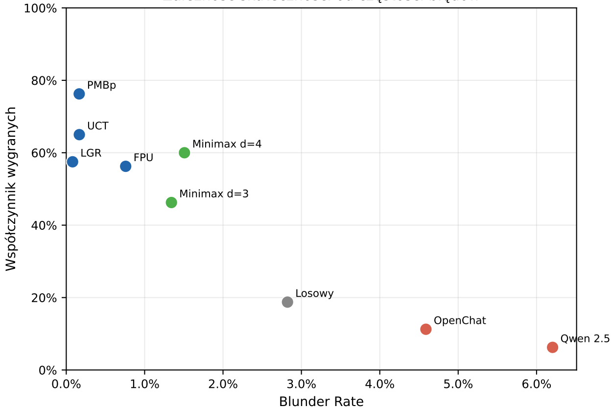
Zależność skuteczności od częstości błędów
