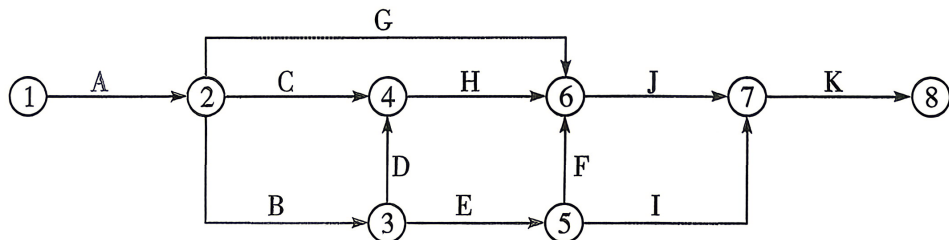
图 6-17 根据表 6-1 绘制的双代号网络图
