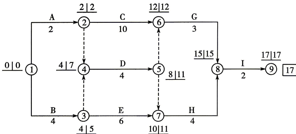
图 6-41 某工程项目网络计划图
