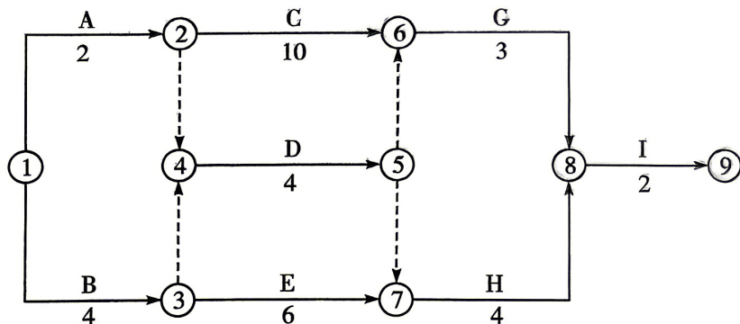
图 6-40 某工程项目网络计划图
