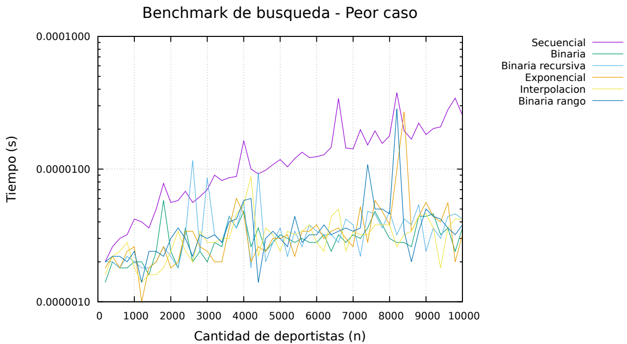
Figura 5.8: Comparación de tiempos en el peor caso
