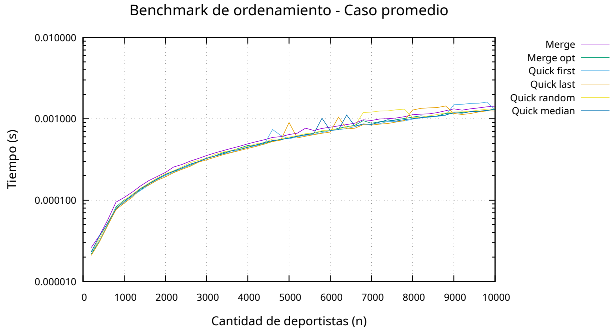
Figura 5.3: Comparación de tiempos en el caso promedio en Divide y Vencerás
