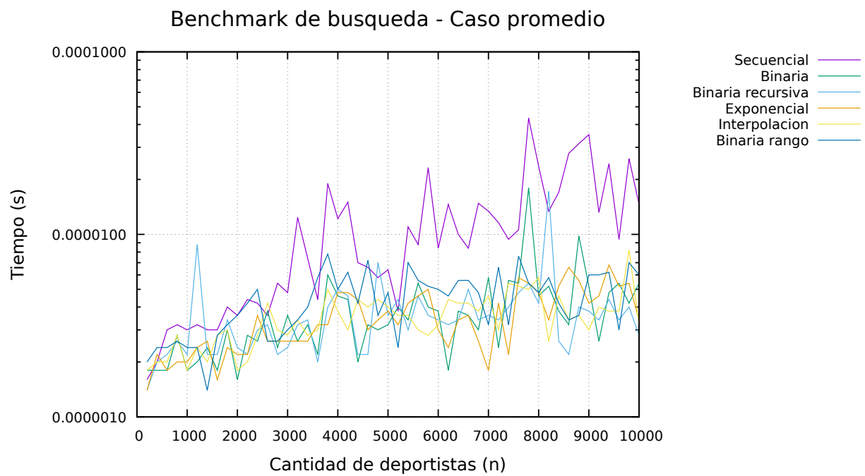
Figura 5.1: Comparación de tiempos en el caso promedio
