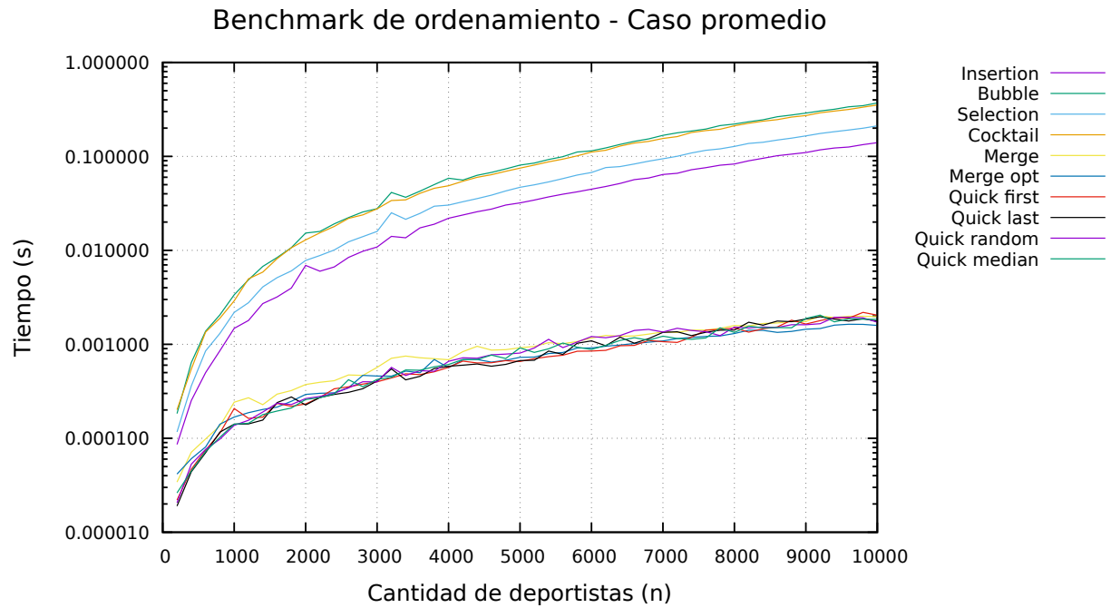
Figura 5.2: Comparación de tiempos en el caso promedio
