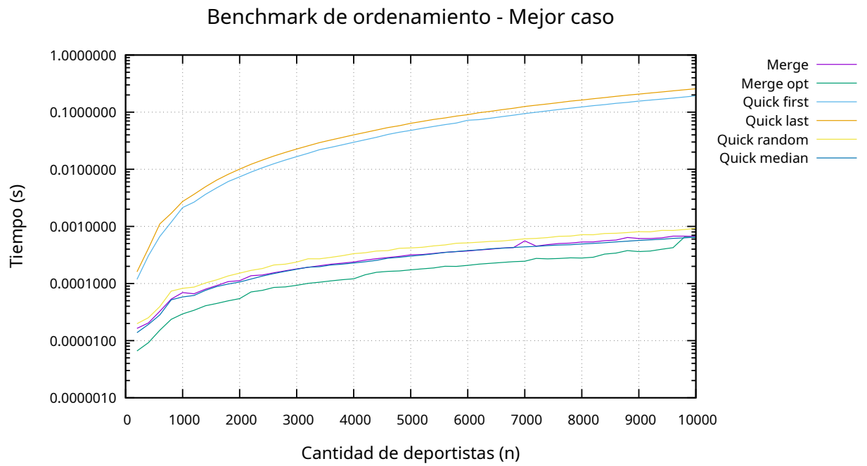
Figura 5.5: Comparación de tiempos en el mejor caso en Divide y Vencerás
