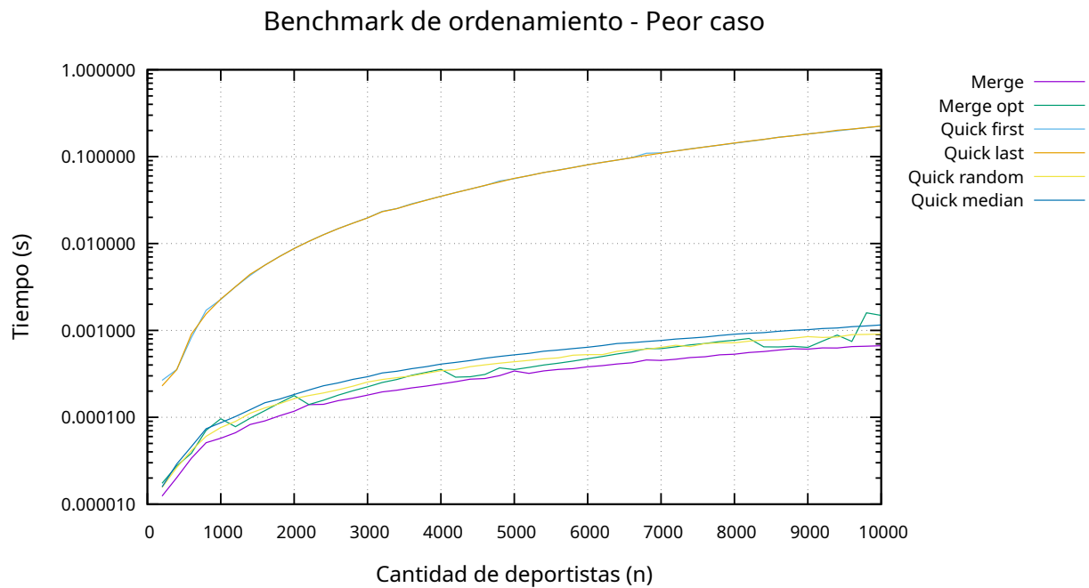
Figura 5.7: Comparación de tiempos en el peor caso en Divide y Vencerás
