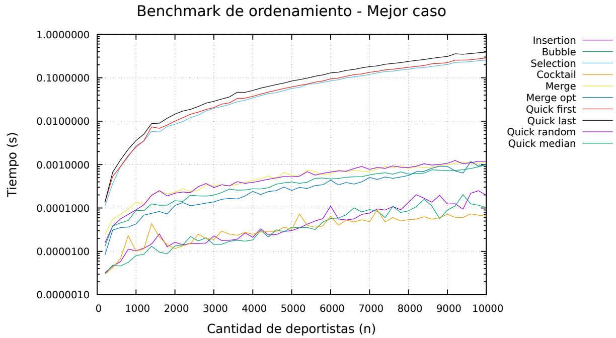
Figura 5.4: Comparación de tiempos en el mejor caso
