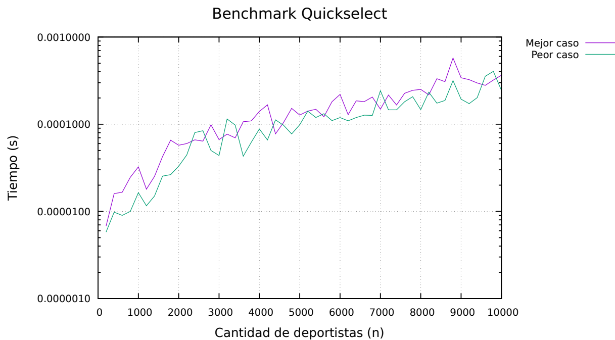
Figura 5.9: Comparación de tiempos en selección
