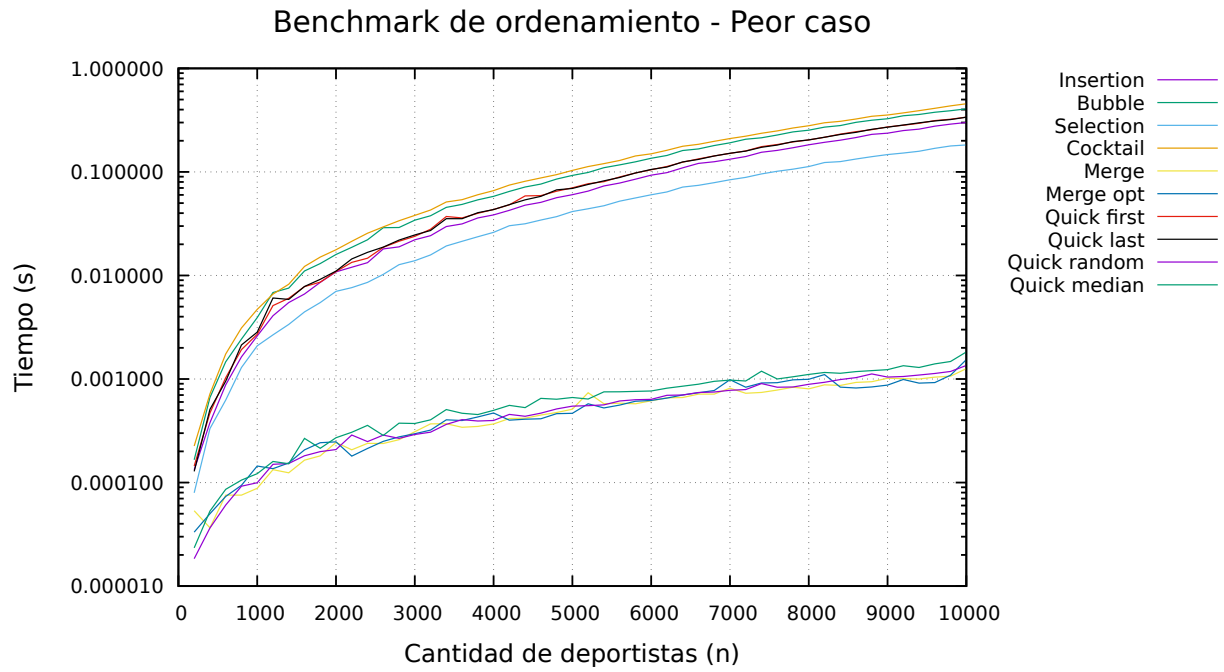
Figura 5.6: Comparación de tiempos en el peor caso
