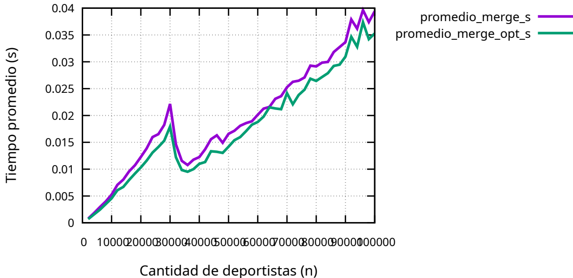
Sort benchmark - caso promedio
