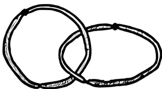
染色体
