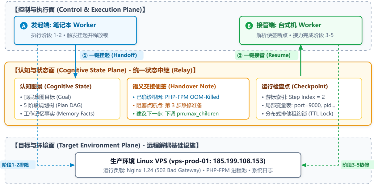
图 1 上下文转移范式 (CHP) 三层解耦架构模型
