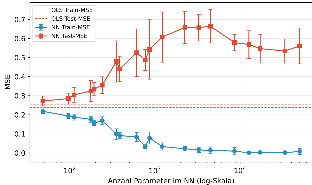
Kapazität vs. Generalisierung: Train- und Test-MSE
