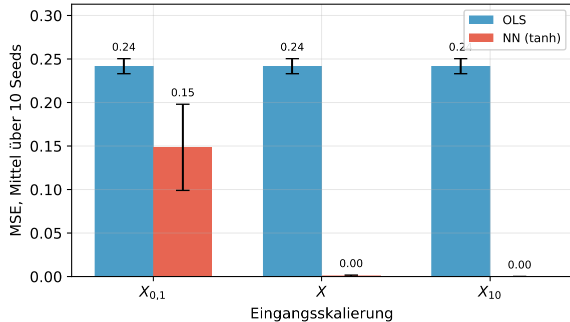
Finaler Train-MSE
