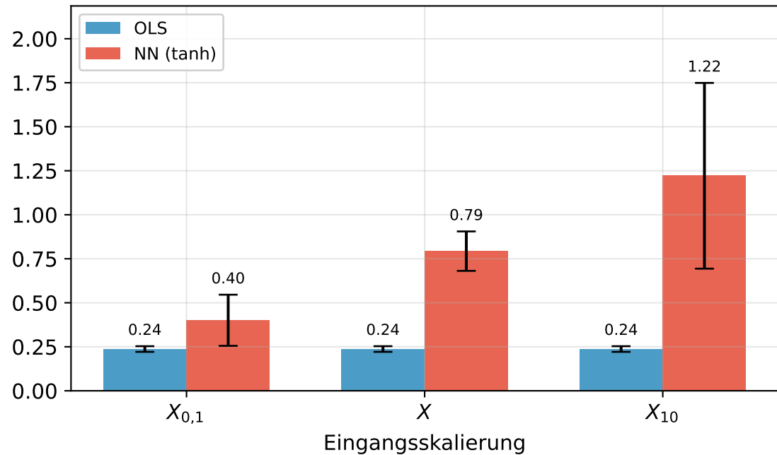
Test-MSE
