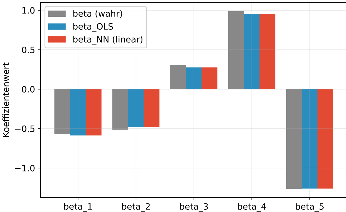
Koeffizienten: wahr vs. OLS vs. lineares NN
